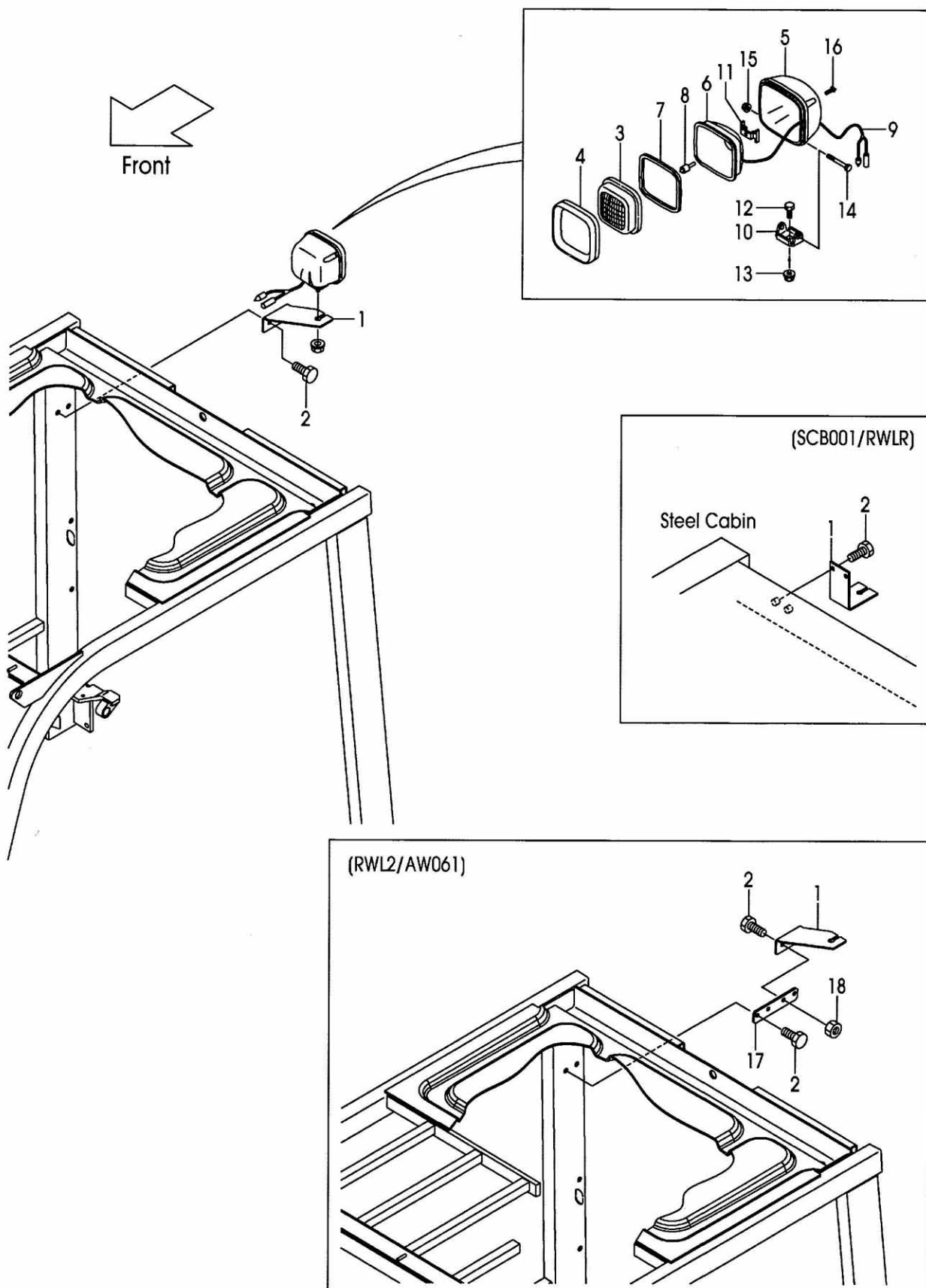
FIG.29 REAR WORKING LIGHT [RWLR] (F7C324P0) リヤワーキングライト
