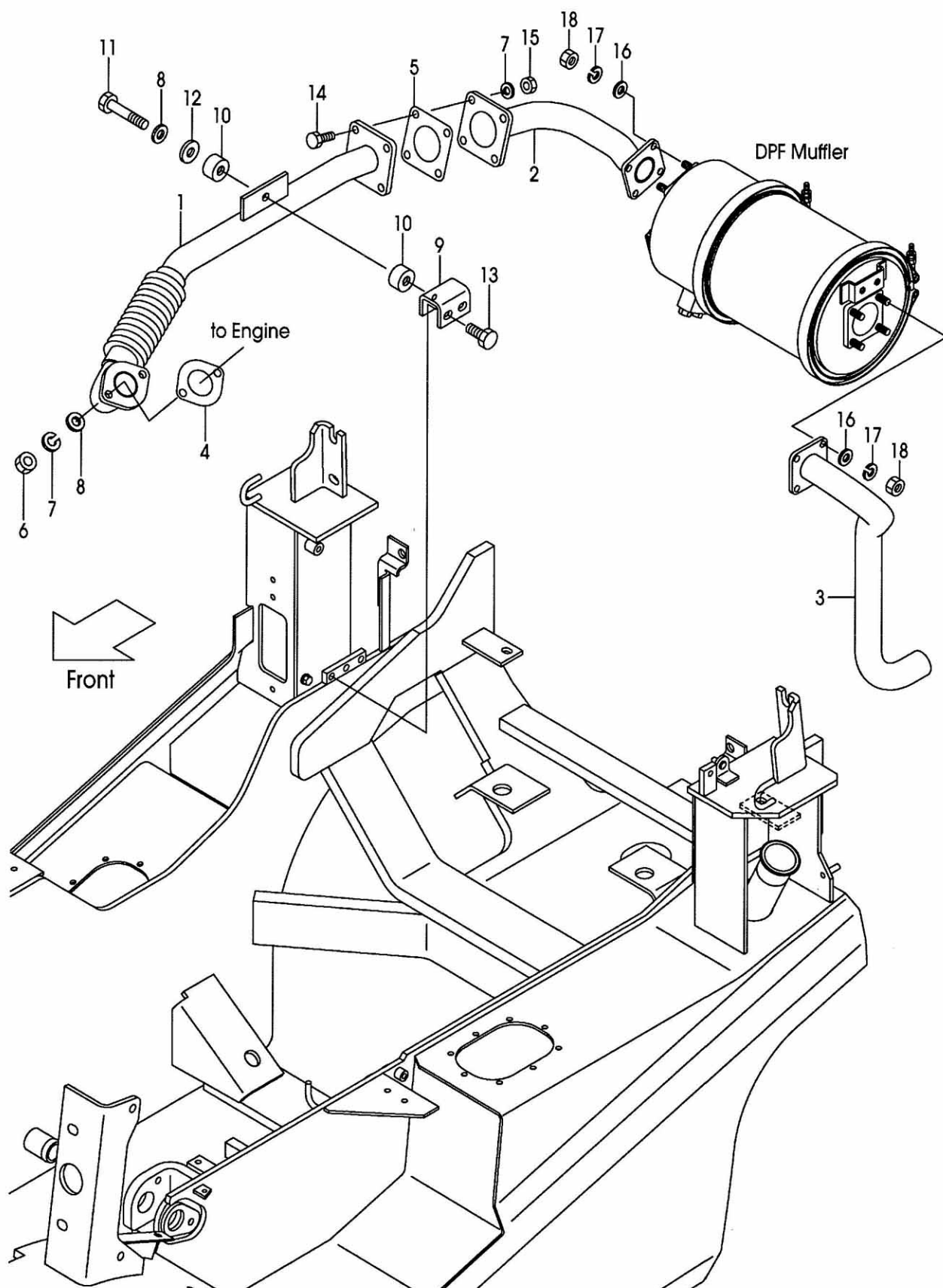
FIG.16 FRONT TUBE & JOINT [DPF] (F7C32390) フロントチューブ&ジョイント
