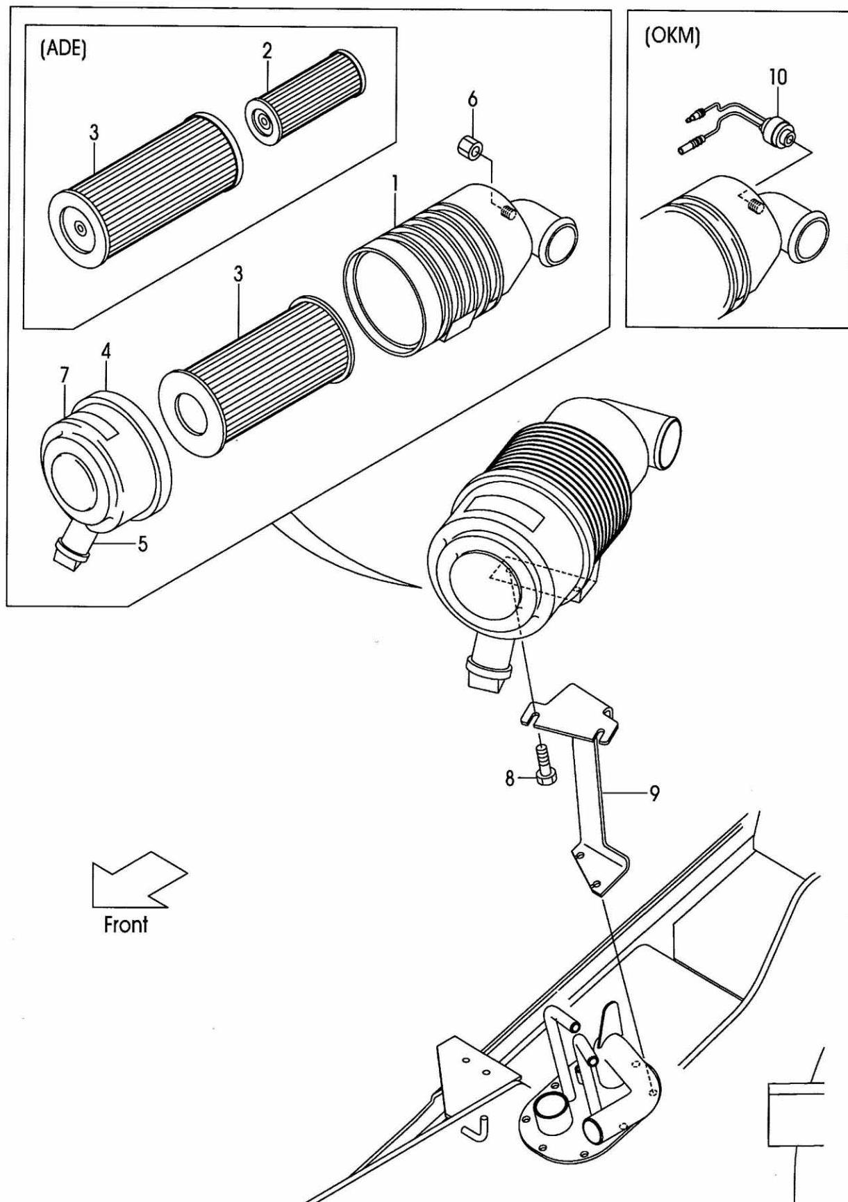
FIG.2 AIR CLEANER (F7C31040) エアークリーナ
