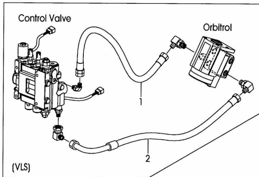
FIG.155 HYDRAULIC LINE (MAIN)(2/4) (F7C37650) ハイドロリックライン(メイン)(2/4)
