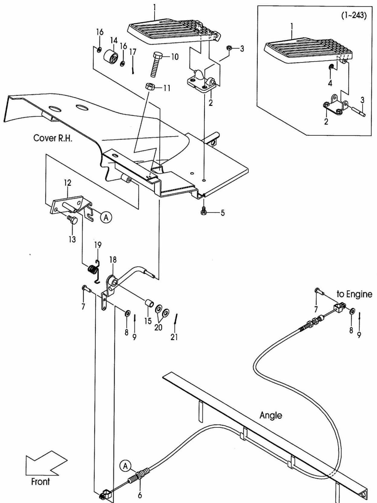
FIG.102 ACCEL PEDAL (F7C35220) アクセルペダル
