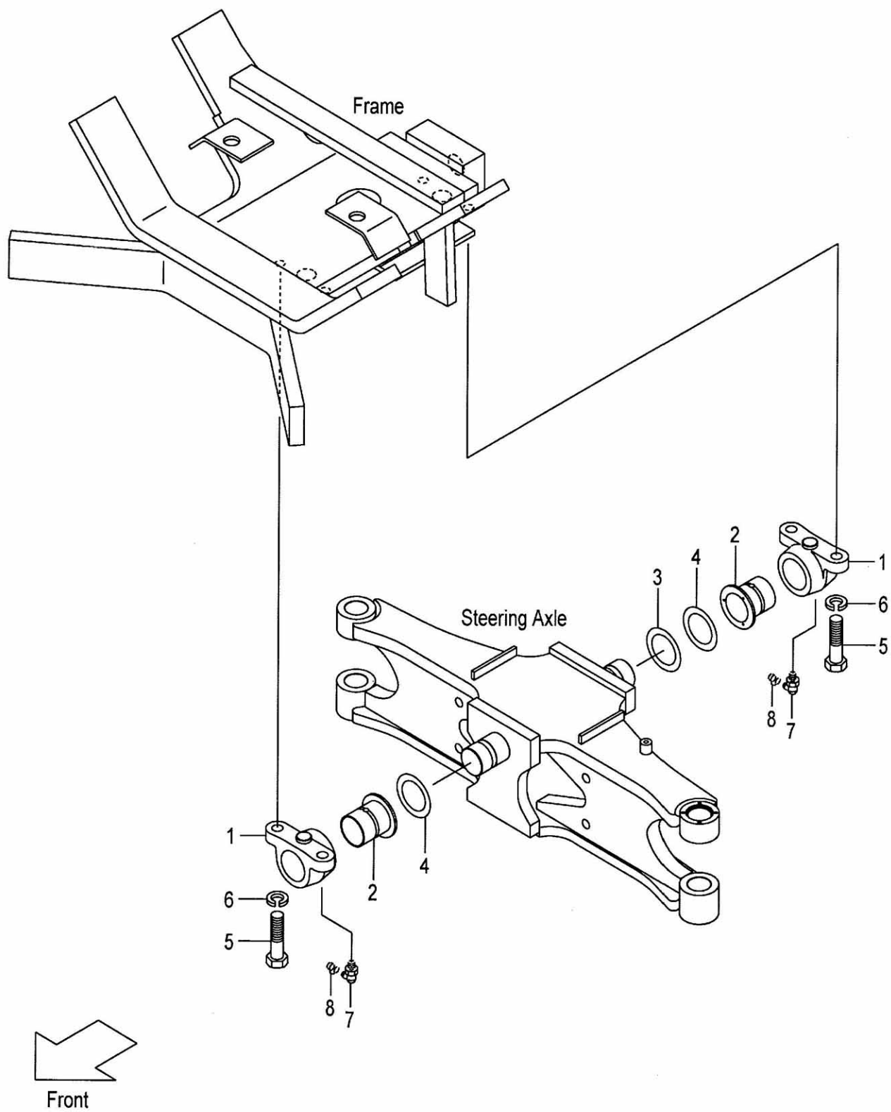
FIG.76 AXLE SUPPORT (F7C34340) アクسلサポート
