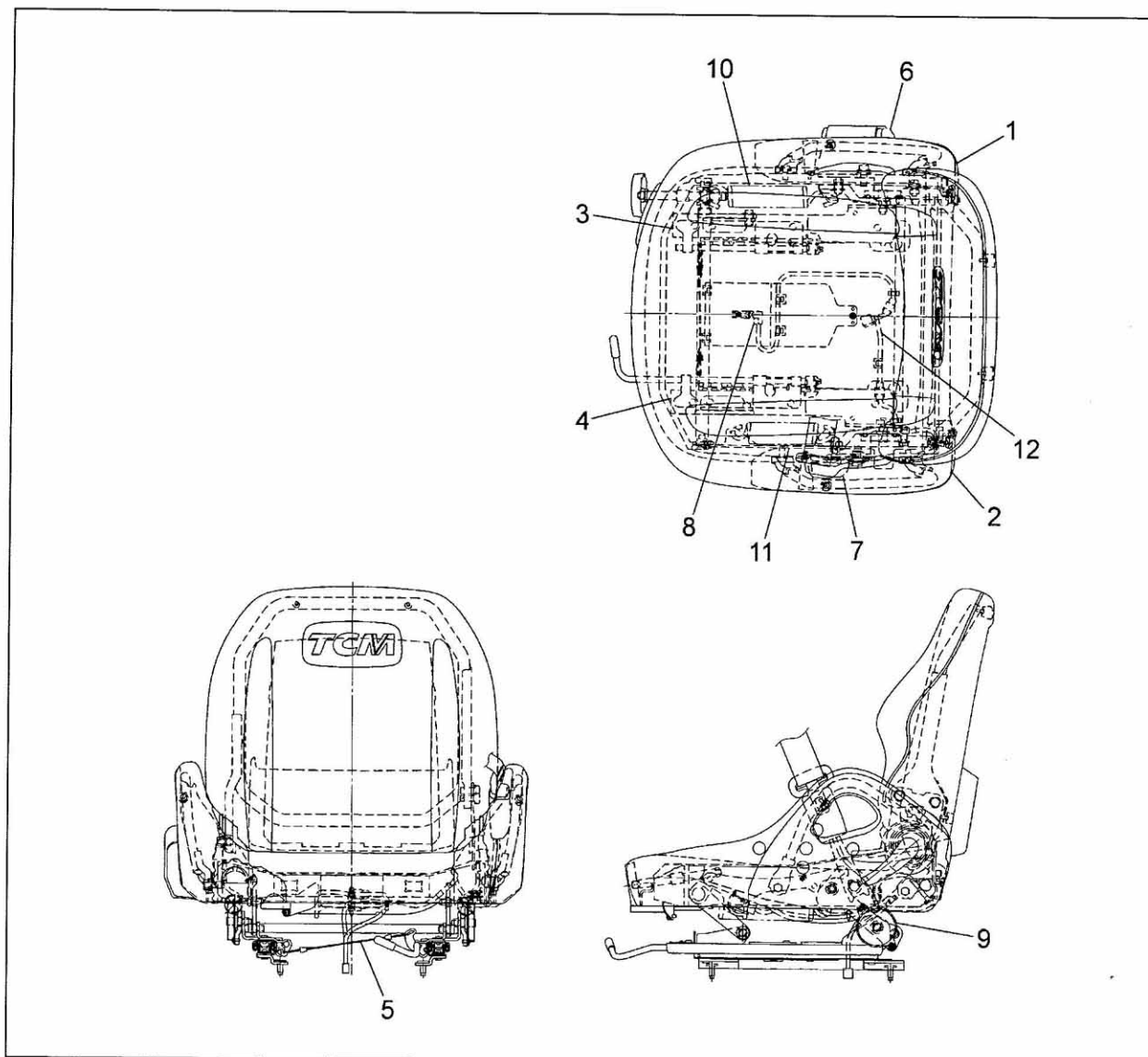
FIG.133 SEAT [OKM/SIL][OKM/EXE][OKM/EXN] (F7C36860) シート
