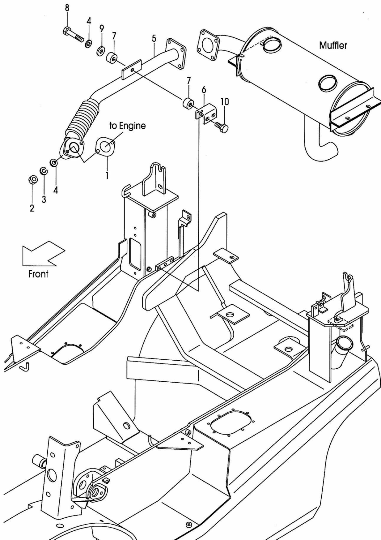
FIG.15 FRONT TUBE & JOINT (F7C32380) フロントチューブ&ジョイント
