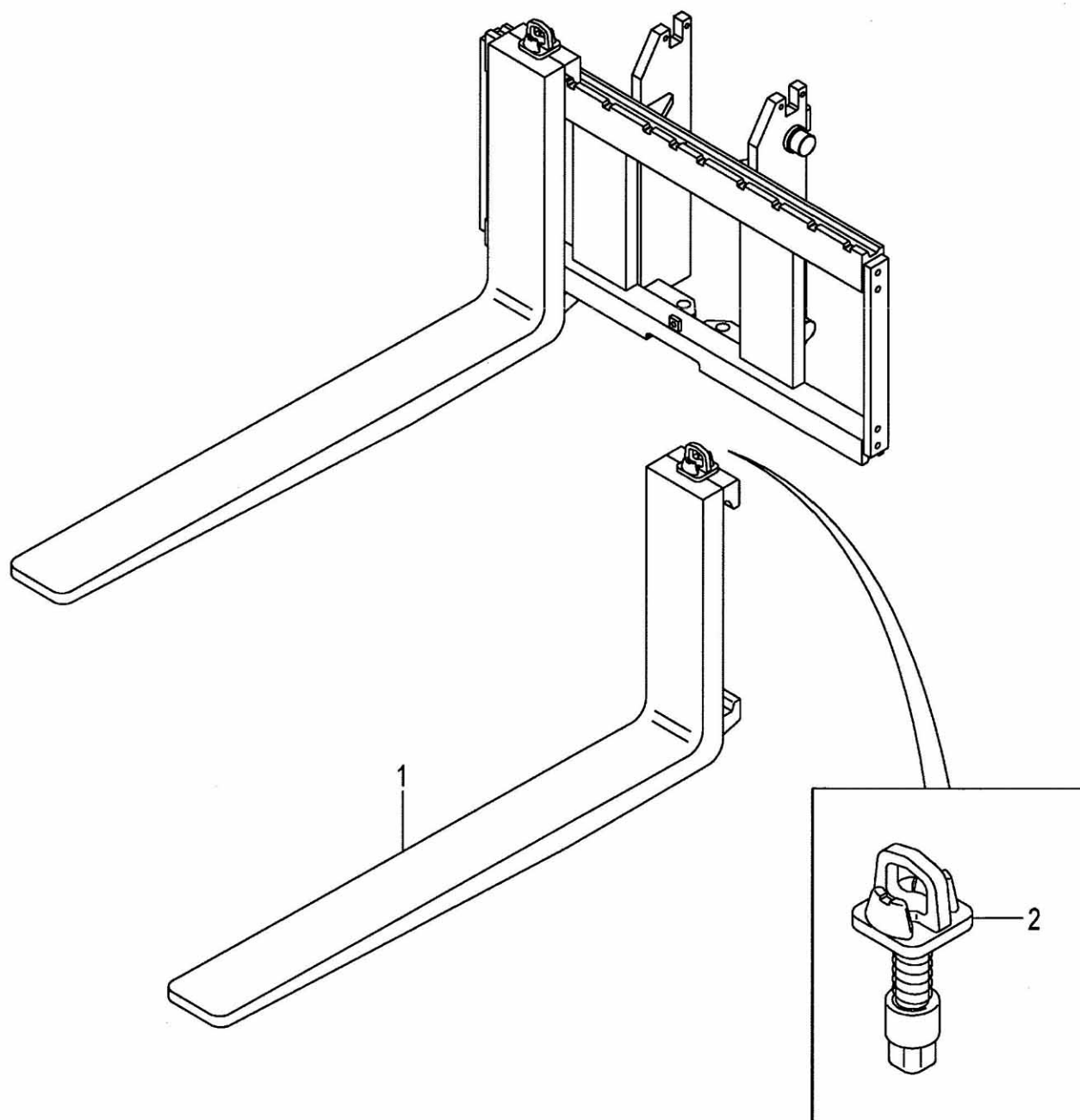
FIG.193 FORK [VFHM2Y5] (M7038130) フォーク
