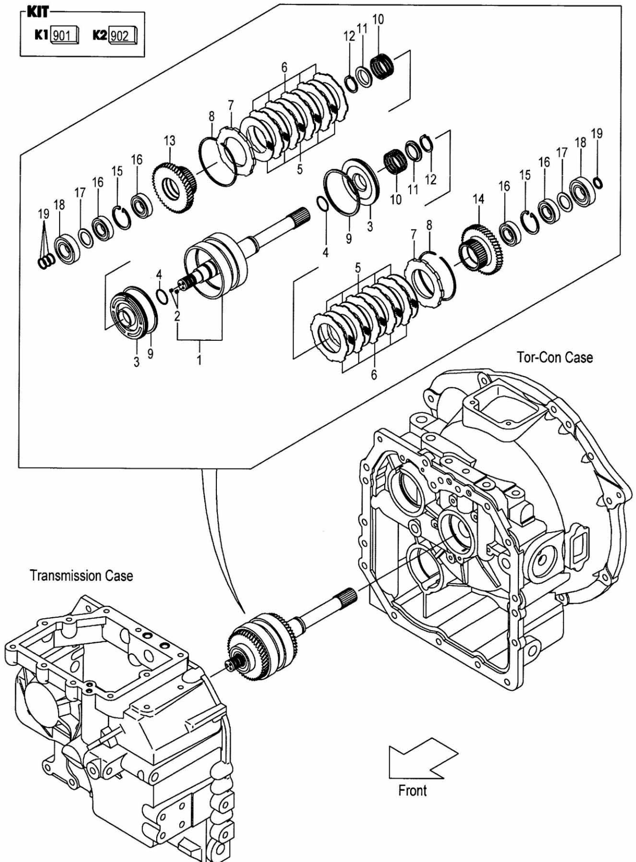
FIG.58 CLUTCH PACK (F7C325B0) クラッチパック
