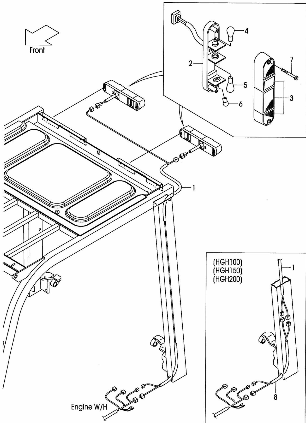
FIG.24 REAR COMBINATION LAMP (F7C324H0) リヤコンビネーションランプ
