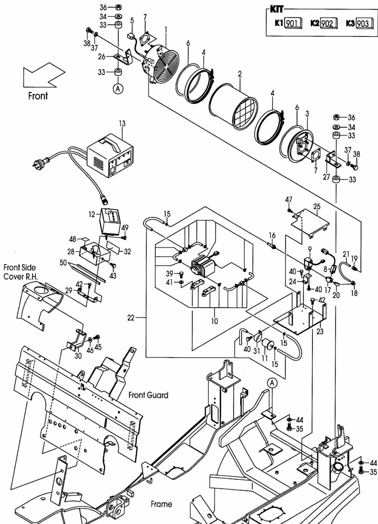
FIG.13 EXHAUST SYSTEM [DPF] (F7C32350) エキゾーストシステム
