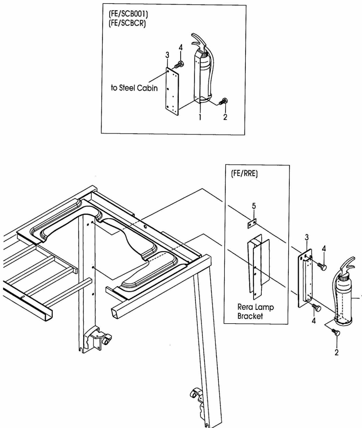
FIG.173 FIRE EXTINGUISHER [FE] (F7C393K0) ファイアクスティング・イッシャ
