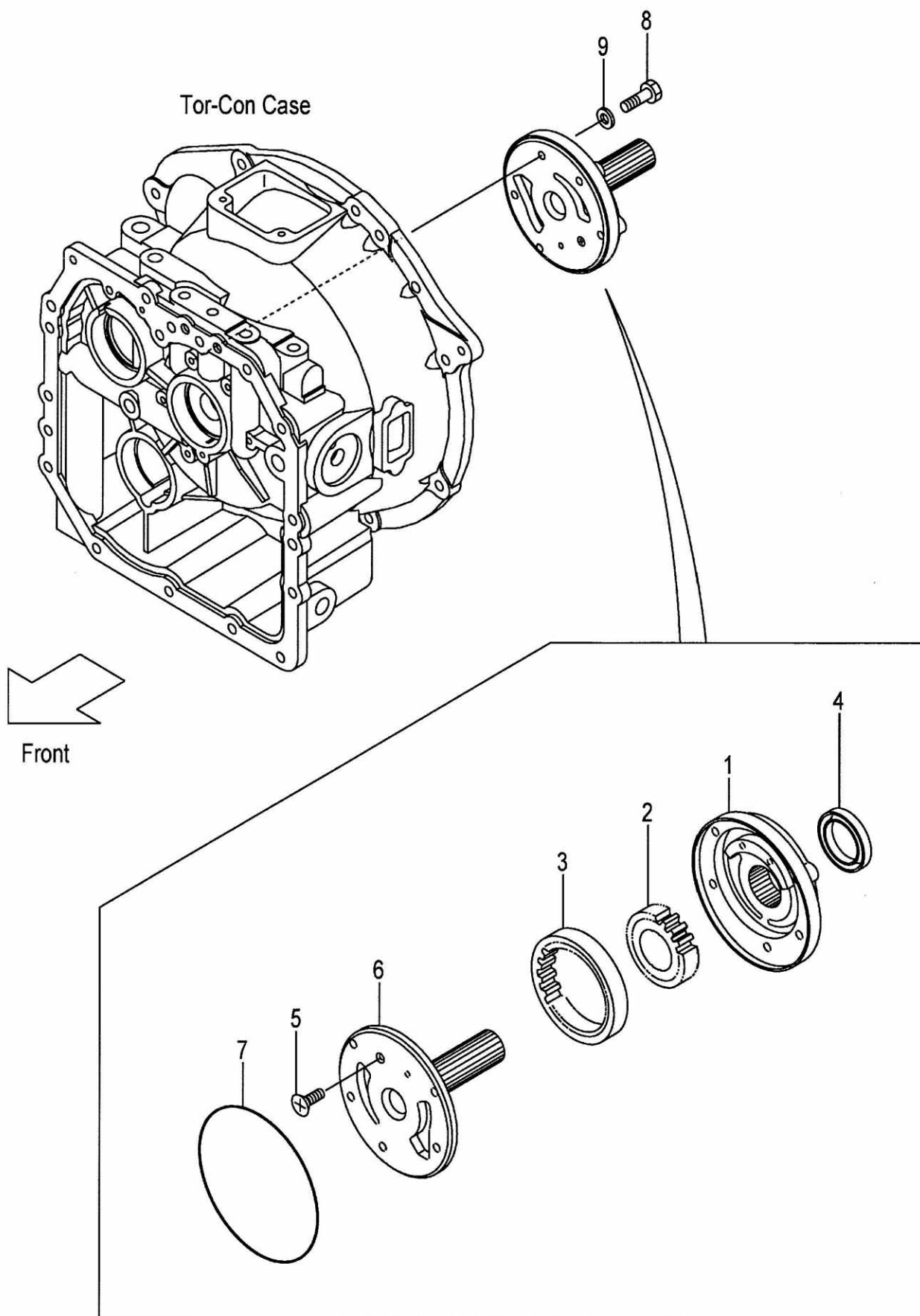
FIG.56 CHARGING PUMP (F7C32590) チャージングポンプ
