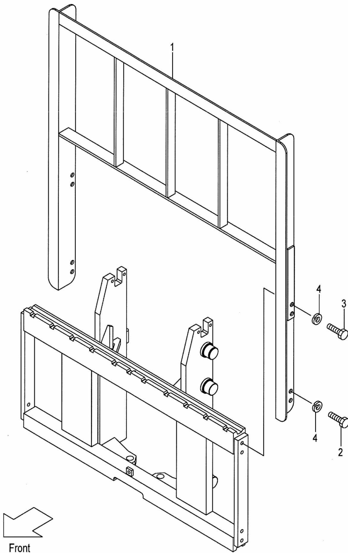
FIG.188 BACKREST [VFM2Y5] (M7038230) バックレスト
