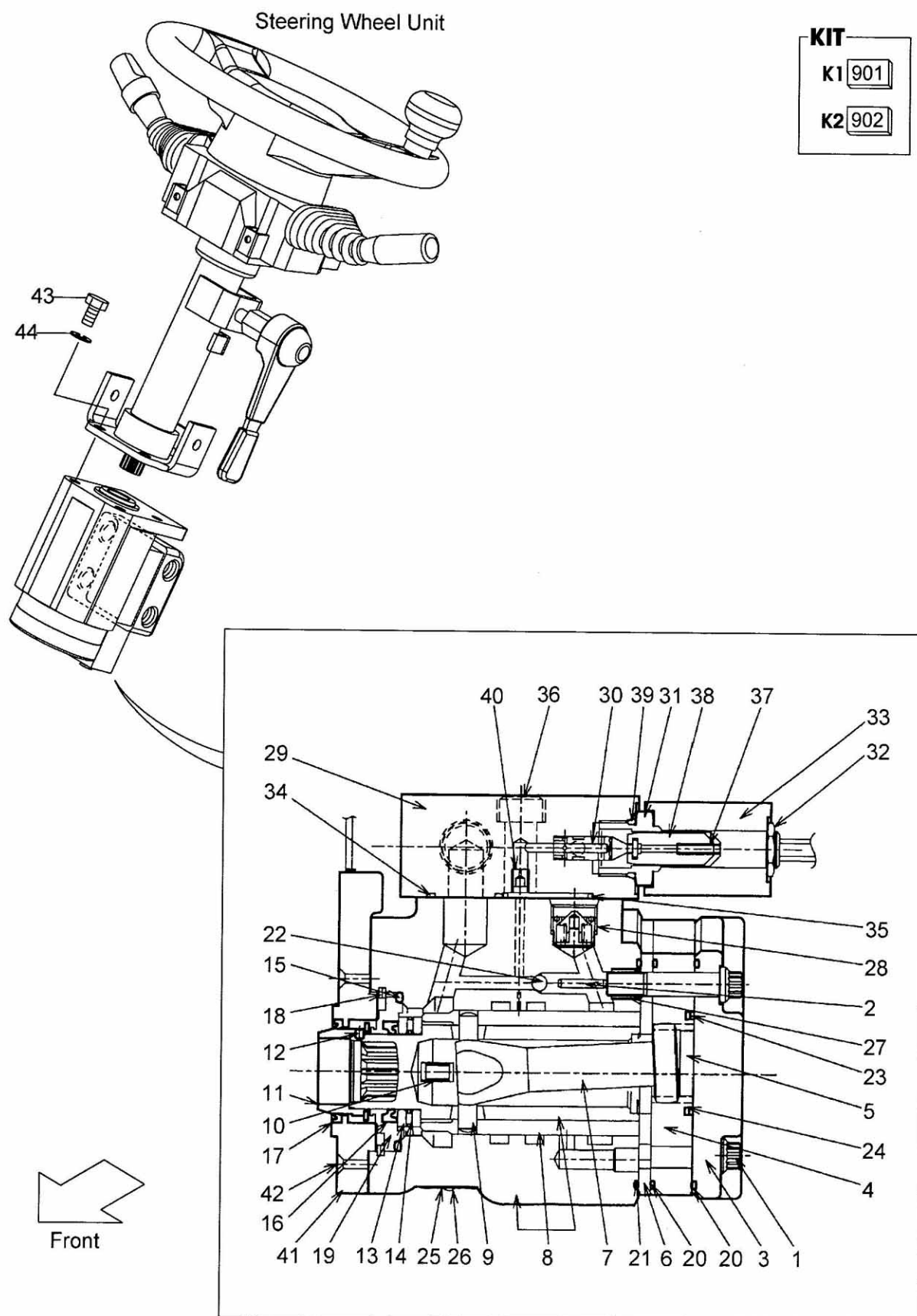
FIG.71 ORBITROL [SRS/EXE][SRS/EXK][SRS/EXN] (F7C34150) オービットロール
