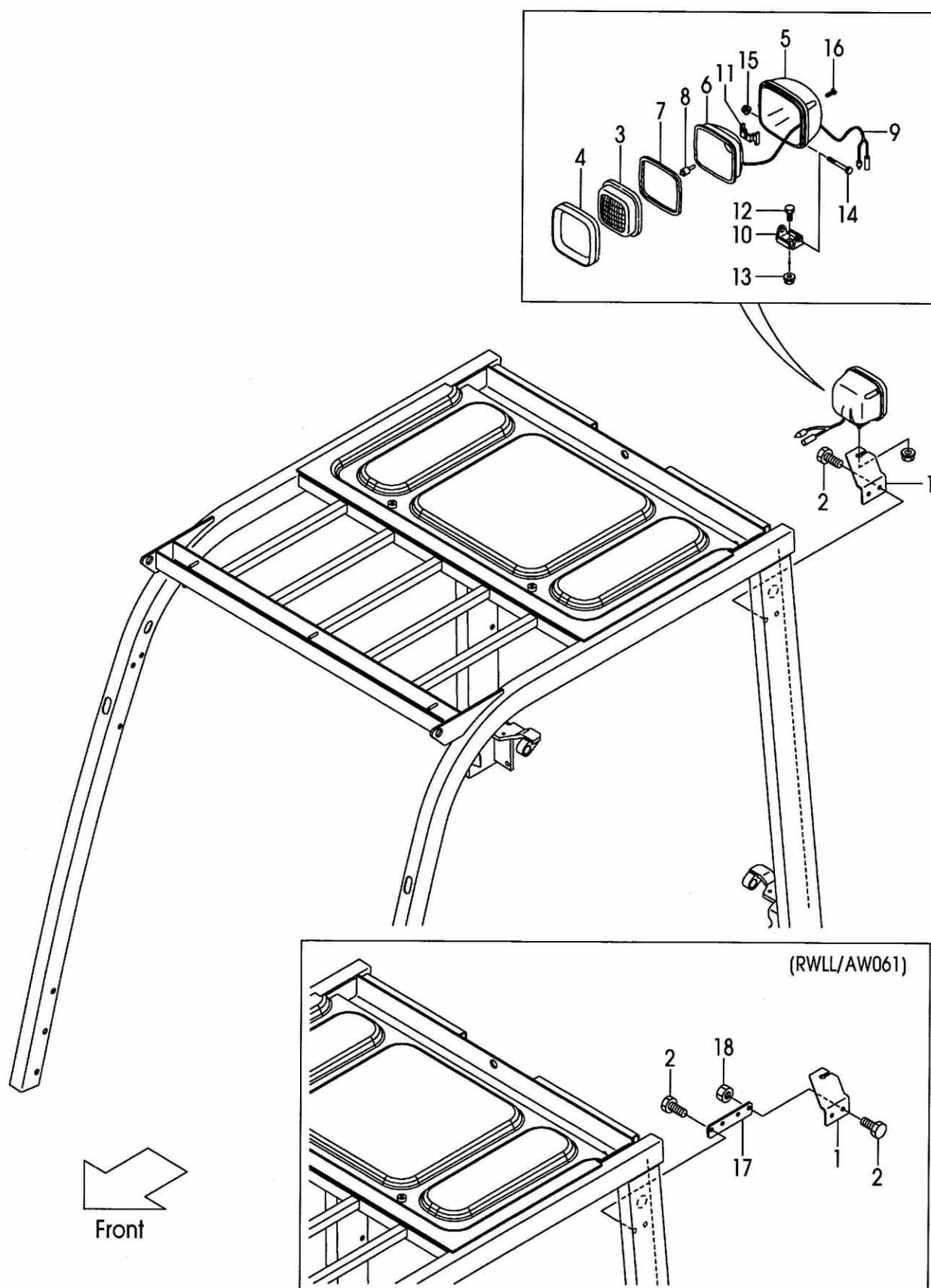
FIG.30 REAR WORKING LIGHT [RWLL] (F7C324Q0) リヤワーキングライト
