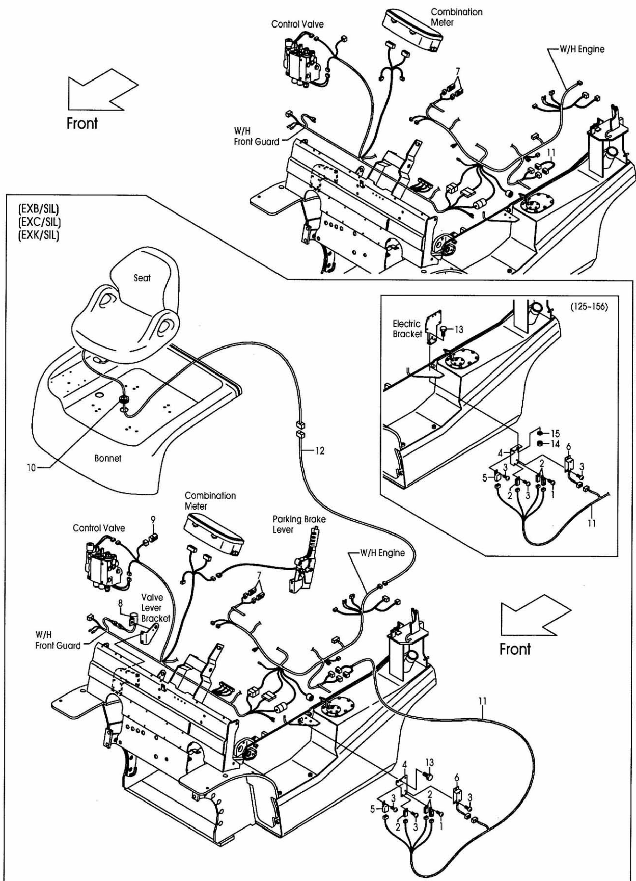
FIG.44 INTERLOCK [EXB][EXC][EXK] (F7C32670) インターロック
