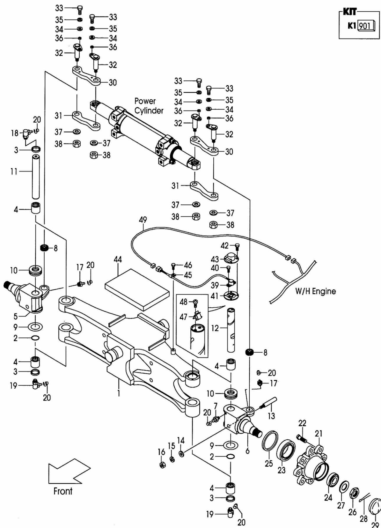
FIG.75 STEERING AXLE [SRS/EXE][SRS/EXK][SRS/EXN] (F7C34330) ステアリングアクスル
