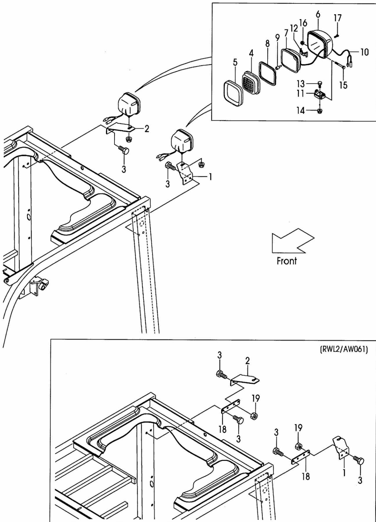
FIG.31 REAR WORKING LIGHT [RWL2] (F7C324R0) リヤワーキングライト
