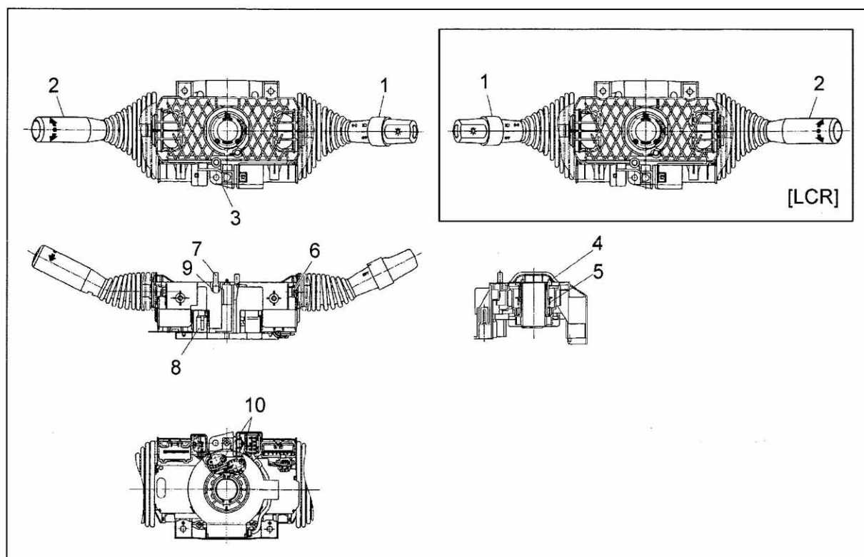
FIG.20 COMBINATION SWITCH (F7C32450) コンビネーションスイッチ
