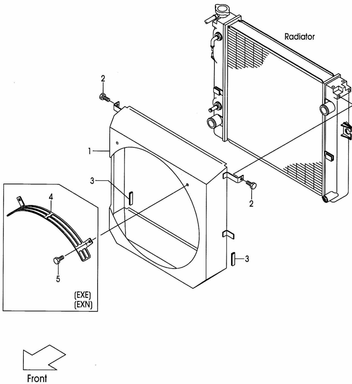
FIG.6 FAN SHROUD (F7C32140) ファンシュラウド
