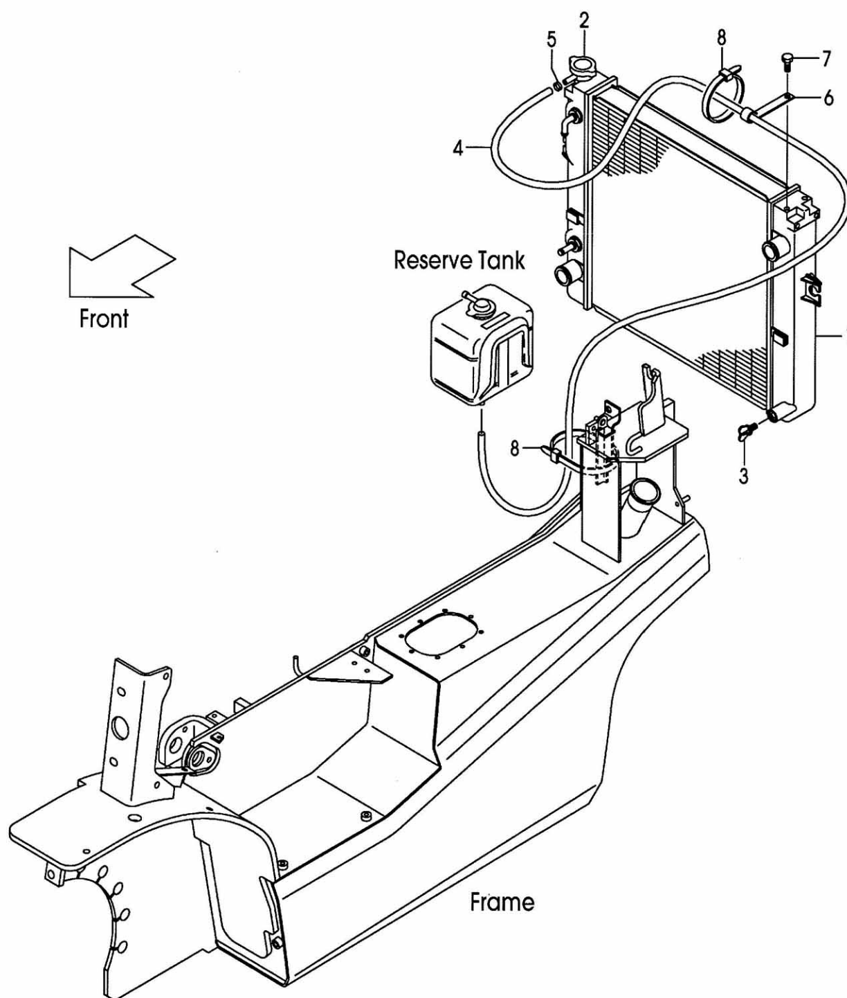
FIG.5 COOLING UNIT (F7C32120) クーリングユニット
