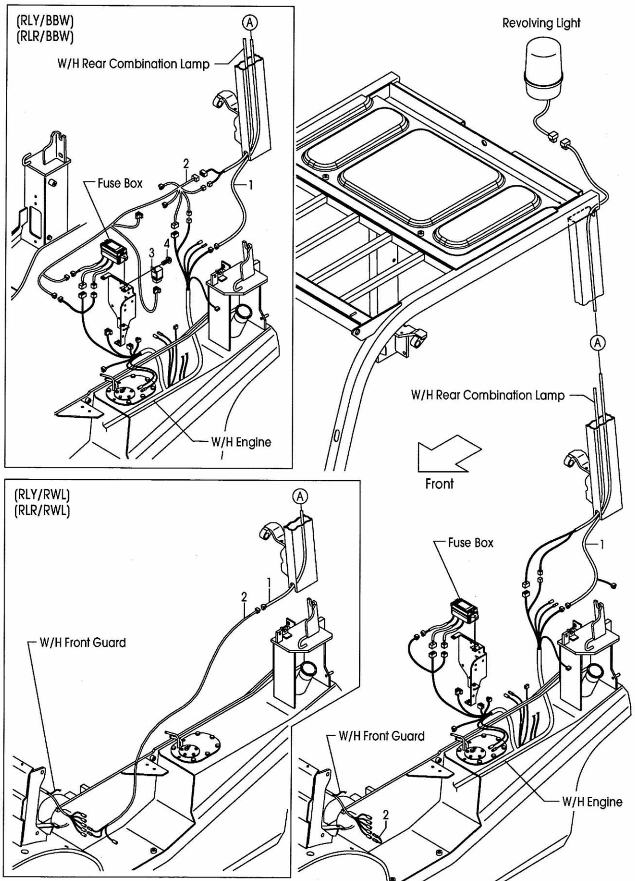
FIG.36 REVOLVING LIGHT WIRE HARNESS [RLY][RLR] (F7C324W0) リボルビングライトワイヤハーネス
