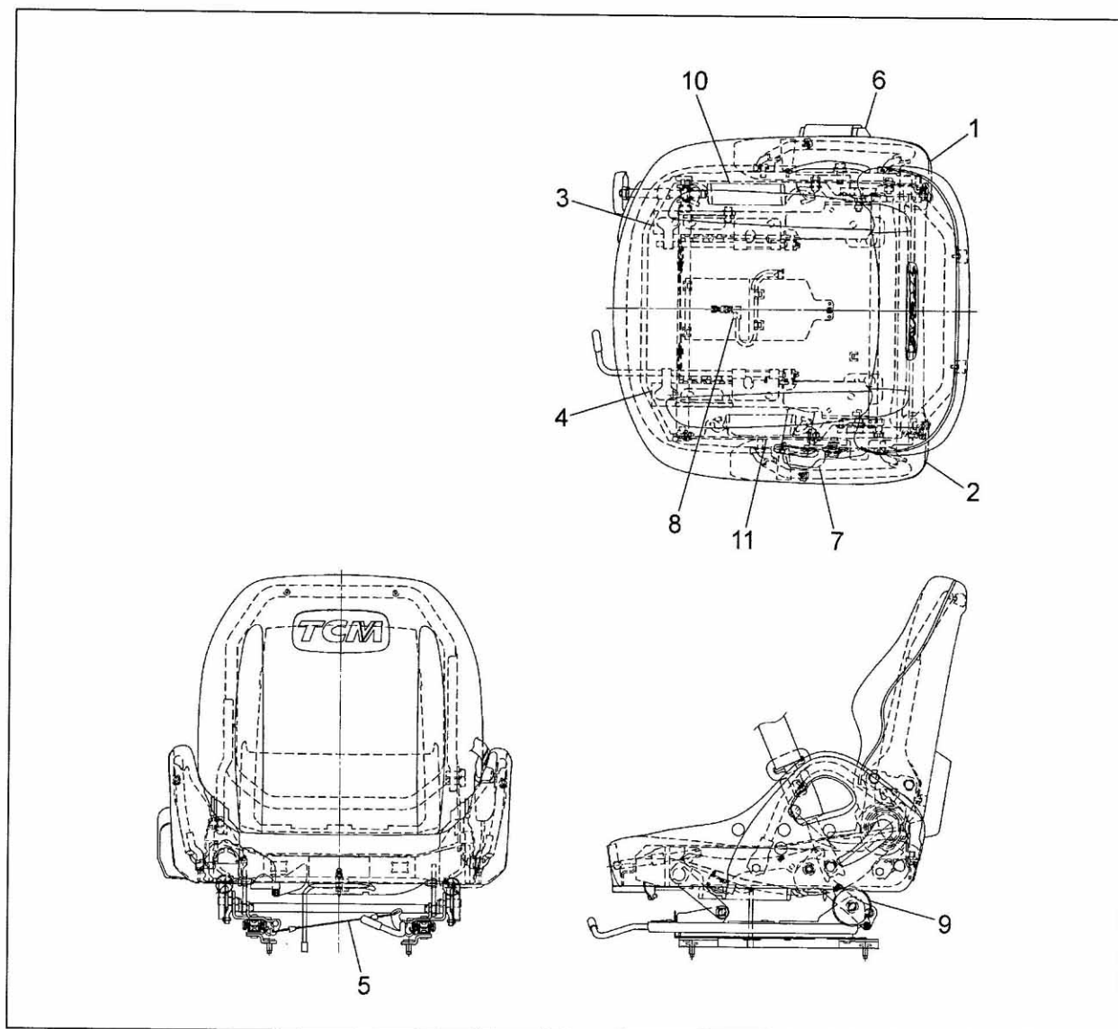
FIG.131 SEAT [SIL][EXE][EXN] (F7C36830) シート
