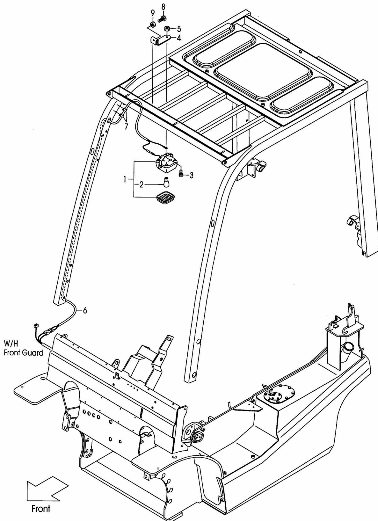
FIG.37 SPOT LIGHT [SPL] (F7C32610) スポットライト
