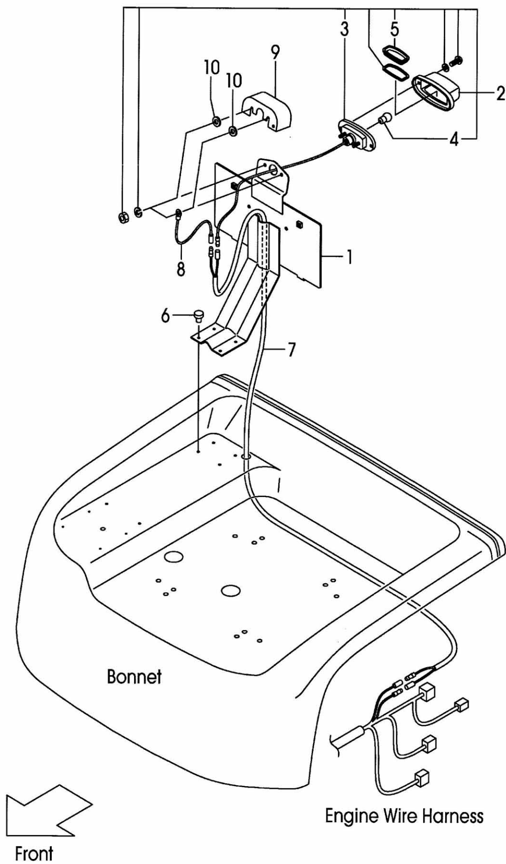
FIG.26 LICENSE LAMP [RRE] (F7C324K0) ライセンスランプ
