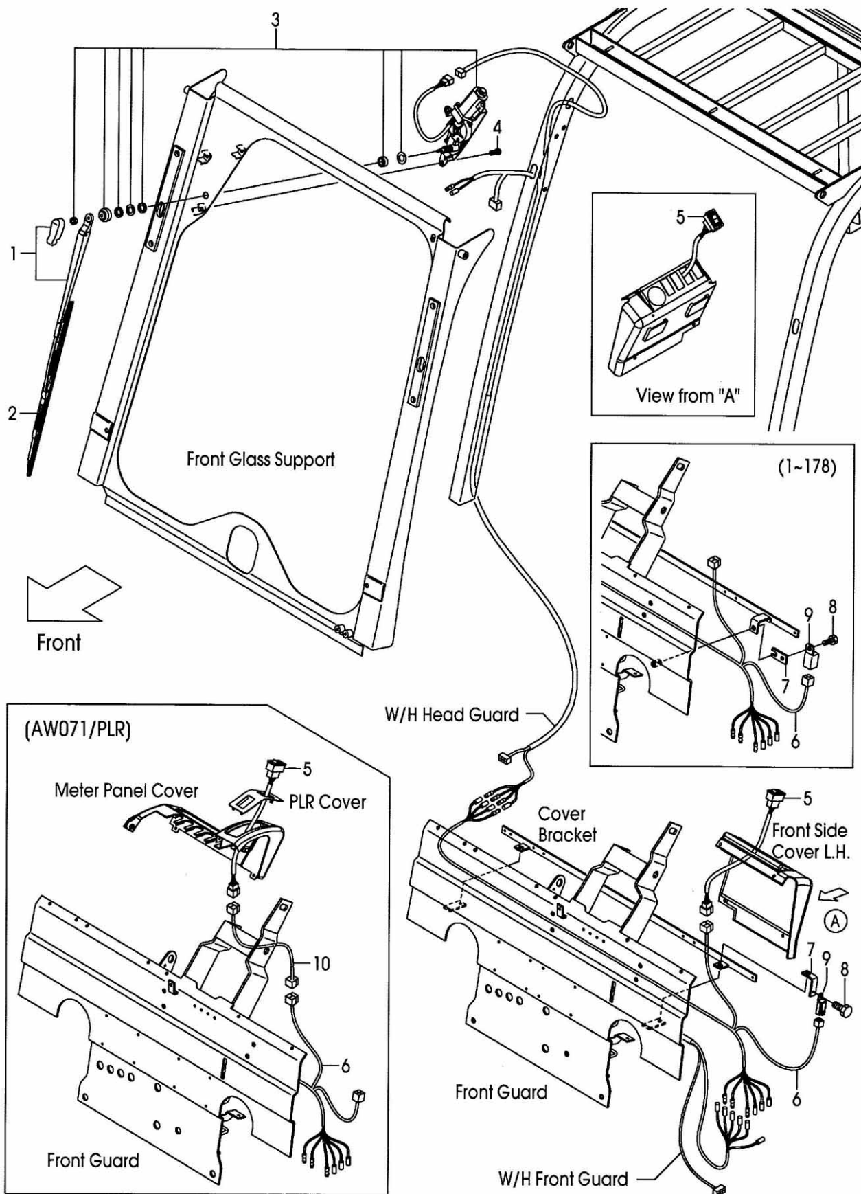
FIG.170 FRONT GLASS WIPER [AW061][AW071] (F7C39320) フロントガラスワイパ°
