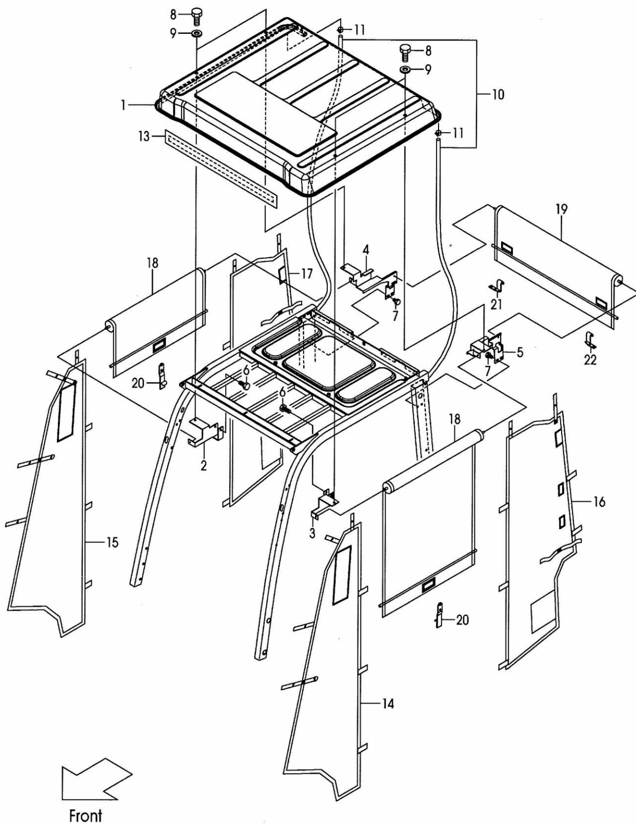
FIG.172 CANVAS CABIN [AW061] (F7C39340) キャンバスキャビン
