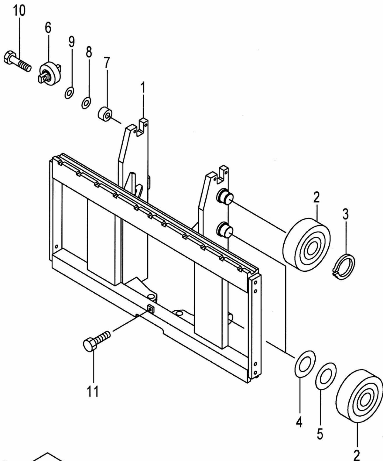
FIG.187 LIFT BRACKET [VFM2Y5] (M7030610) リフトブラケット
