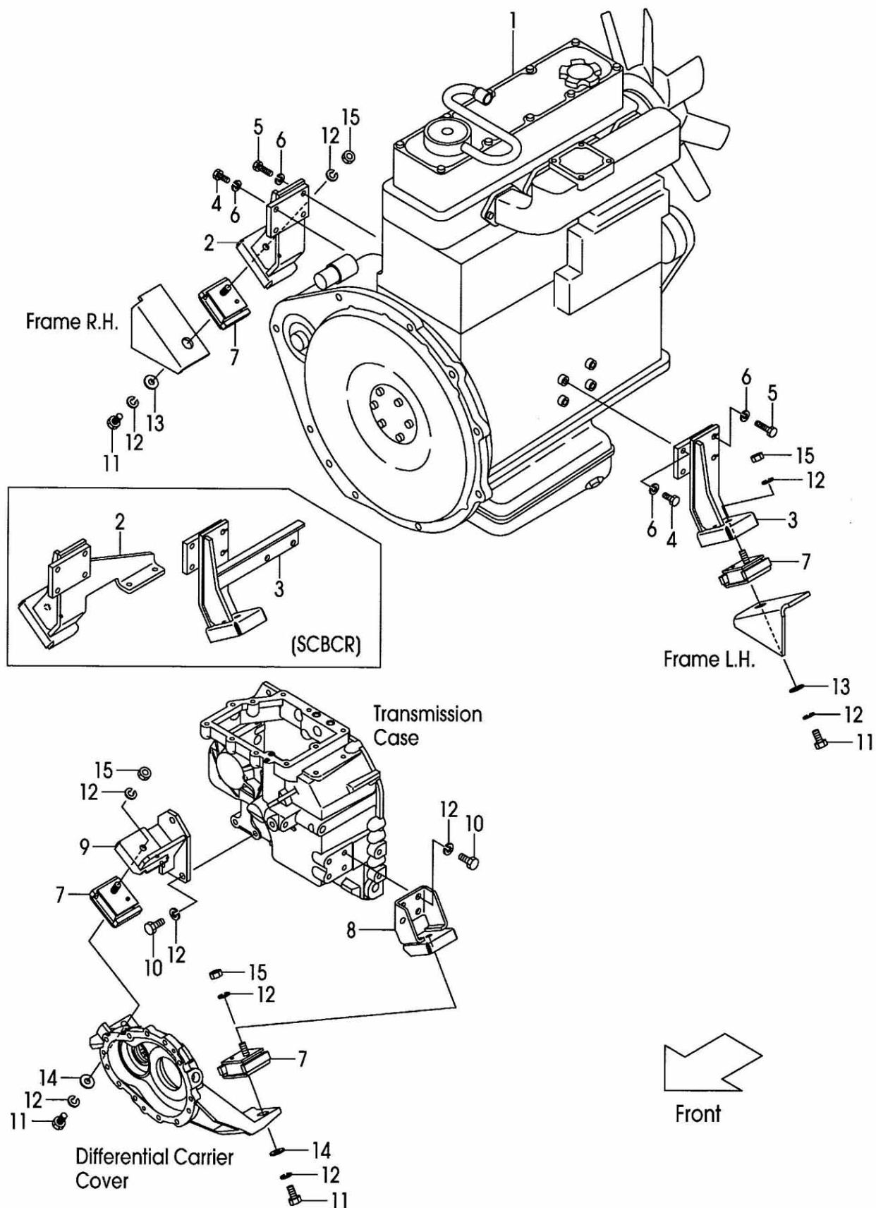
FIG.1 ENGINE MOUNT (F7C31020) エンジンマウント
