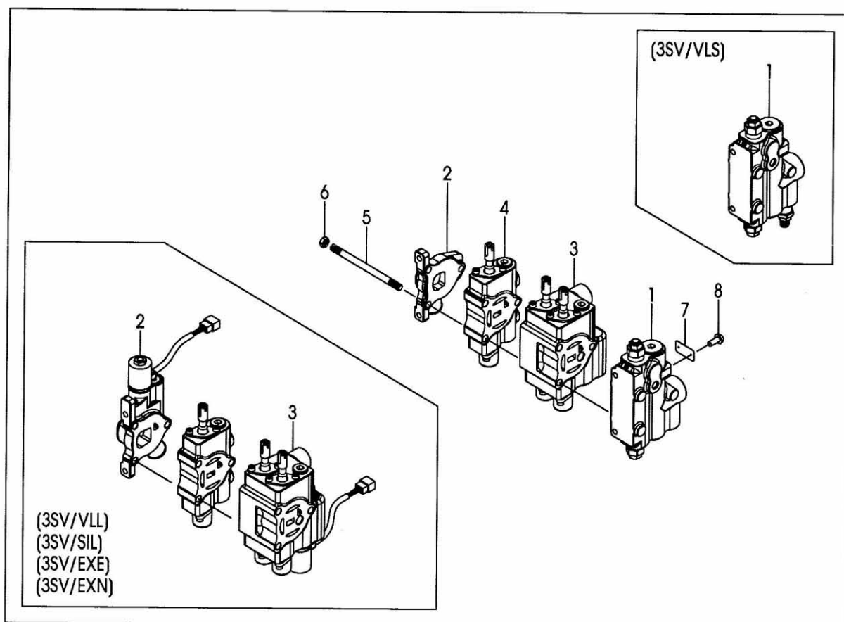
FIG.141 CONTROL VALVE [3SV] (F7C37320) コントロールバルブ
