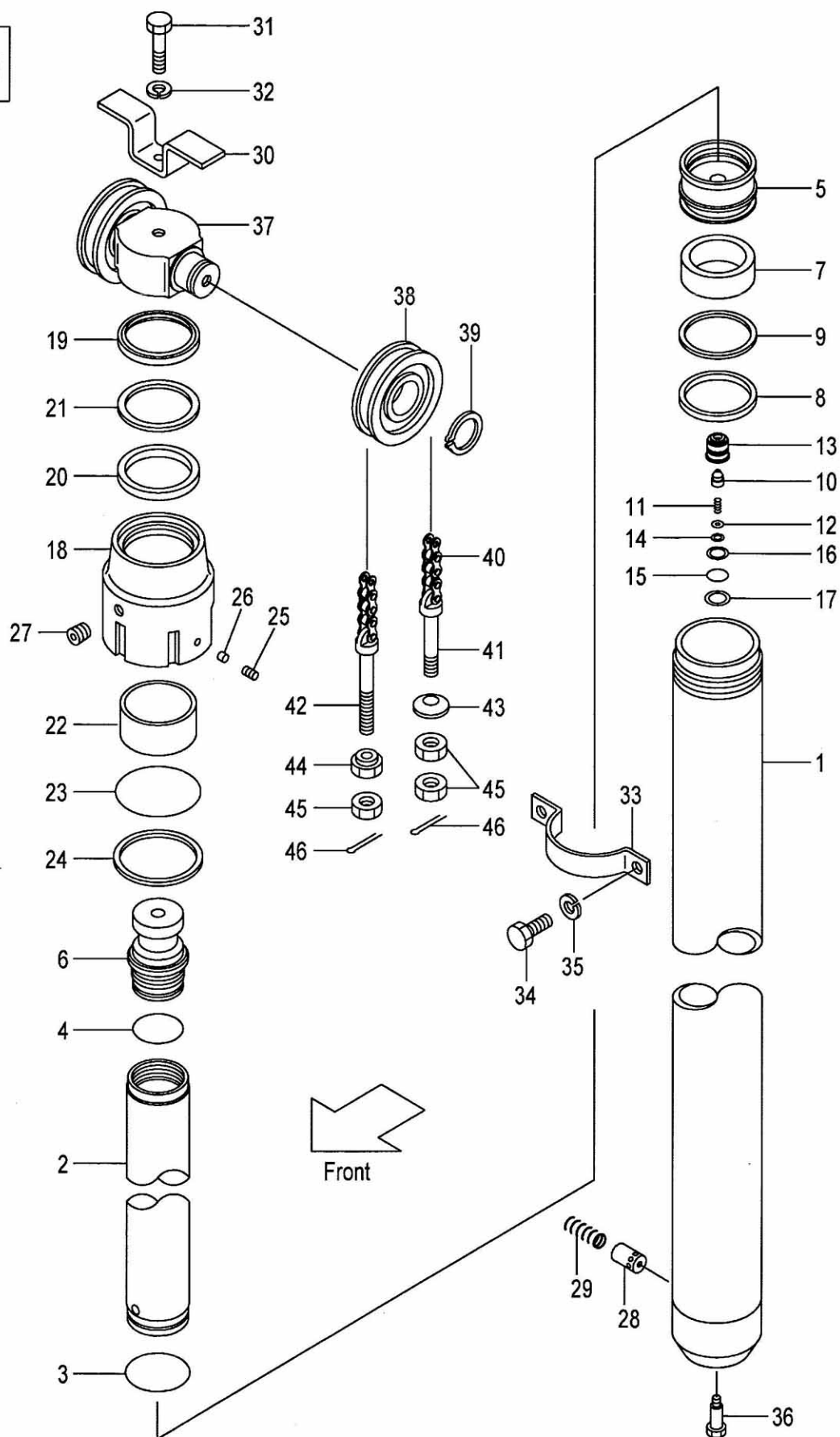
FIG.197 LIFT CYLINDER(FRONT) [VFHM2Y5] (M7030810) リフトシリンダ(フロント)
