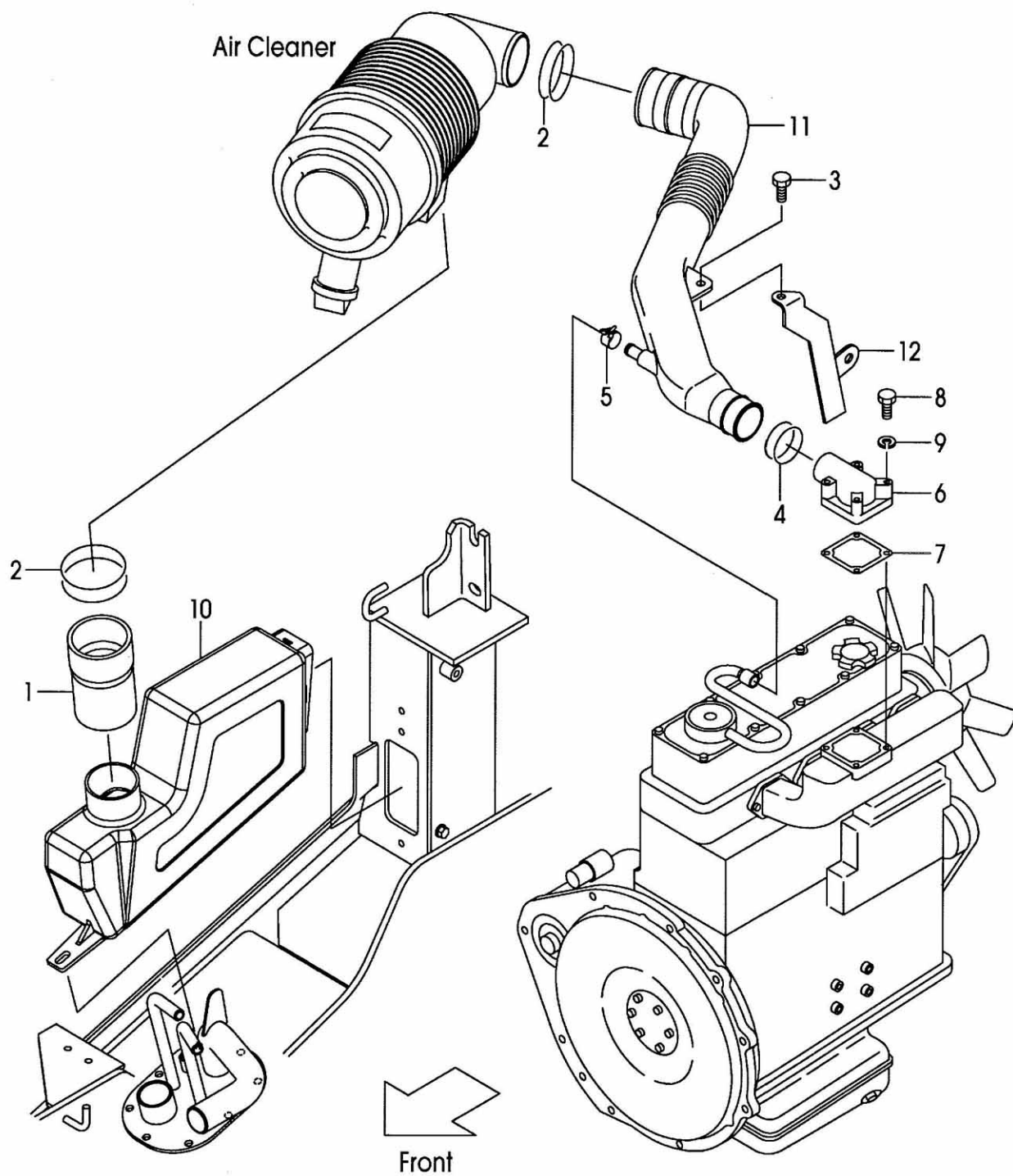
FIG.3 AIR DUCT (F7C31060) エアダクト
