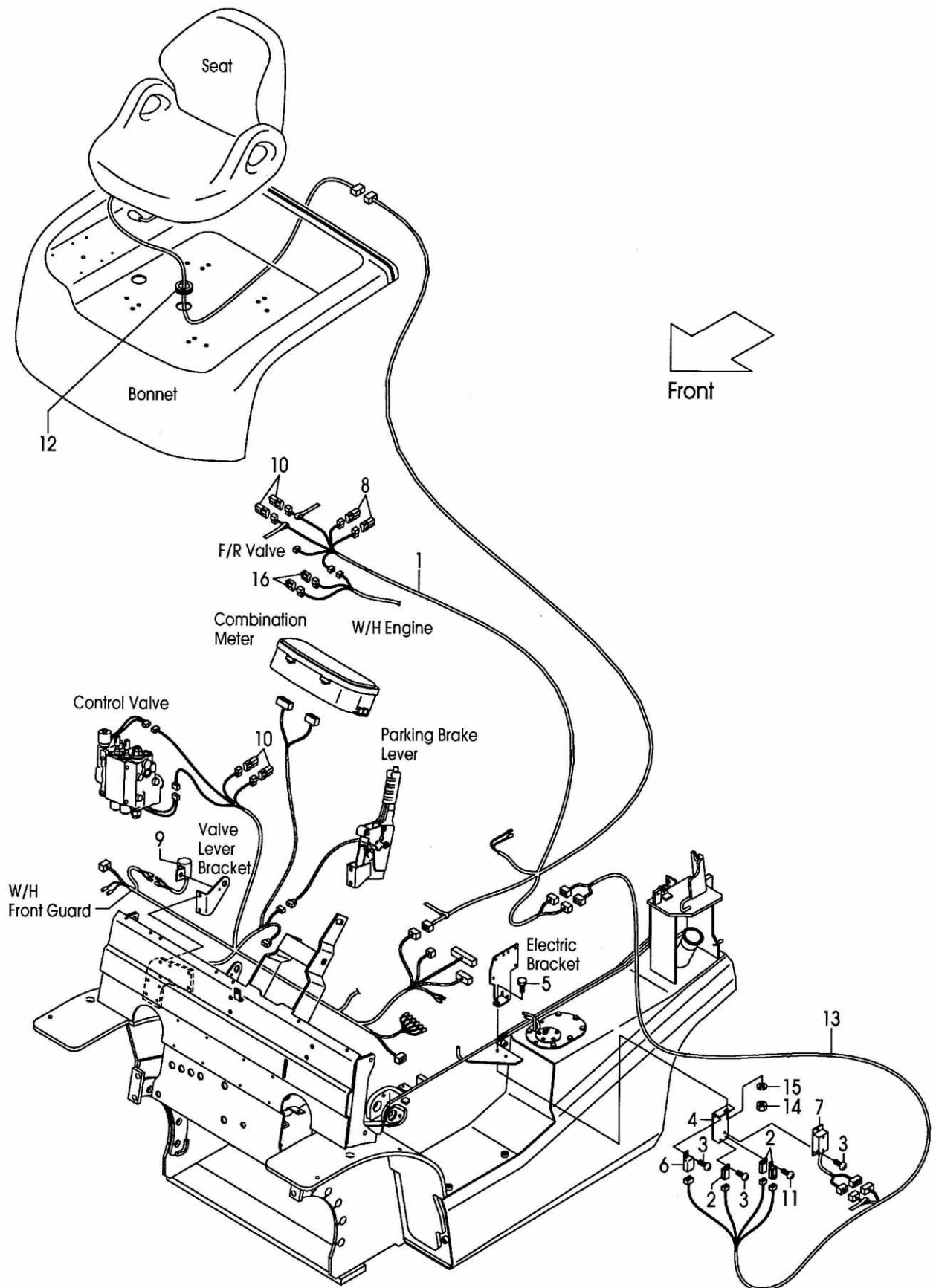
FIG.43 INTERLOCK [SIL][EXE][EXN] (F7C32650) インターロック
