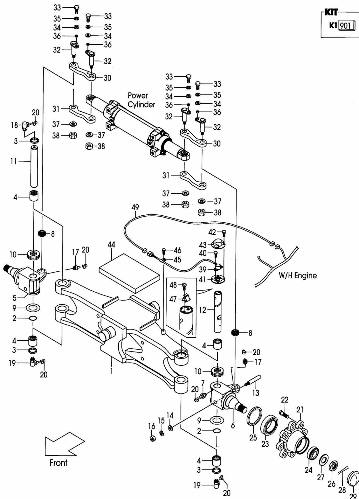
FIG.73 STEERING AXLE (F7C34310) ステアリングアクスル
