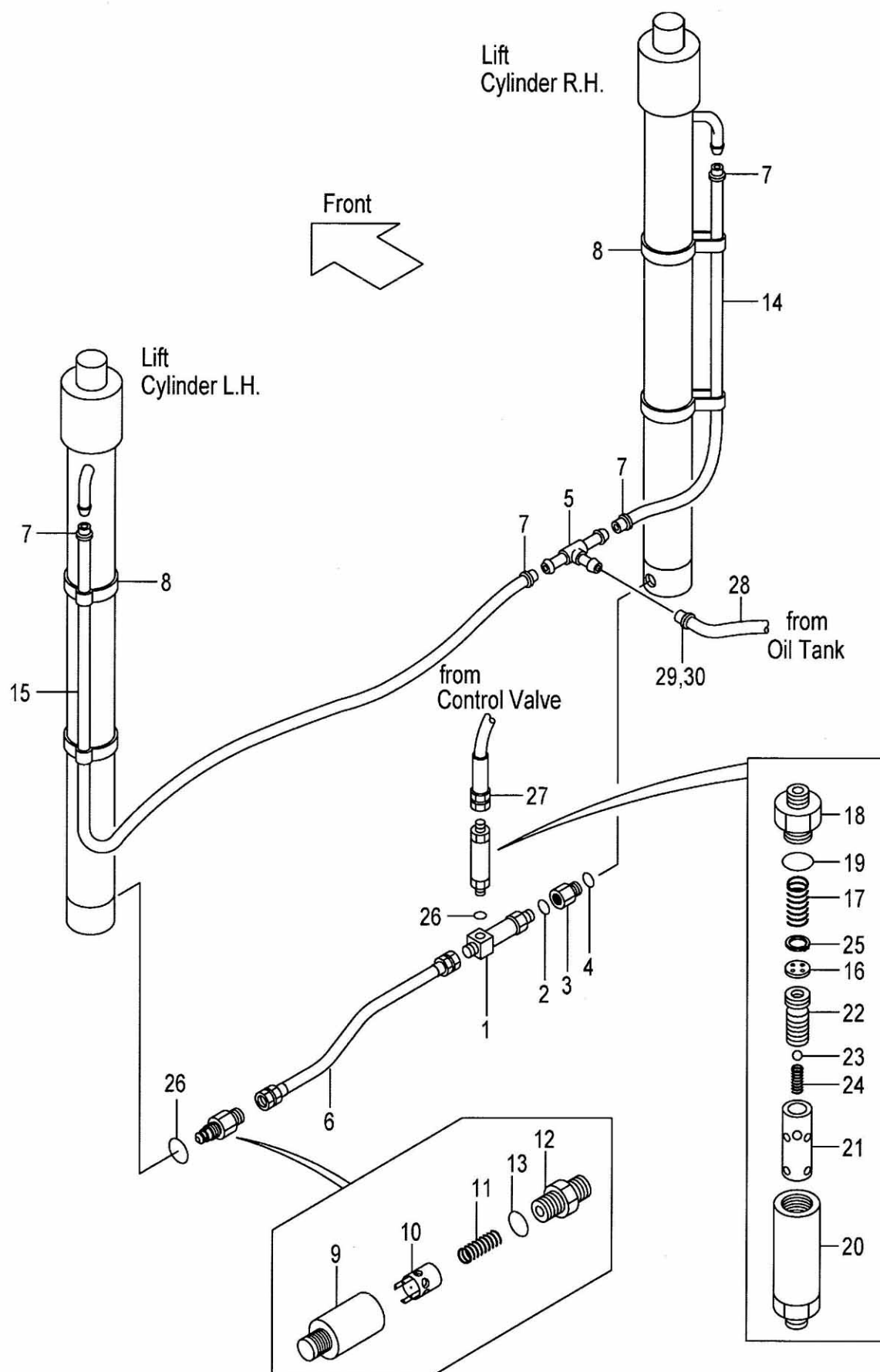
FIG.185 MAST PIPING [VM2Y5] (M7038420) マストパイピング
