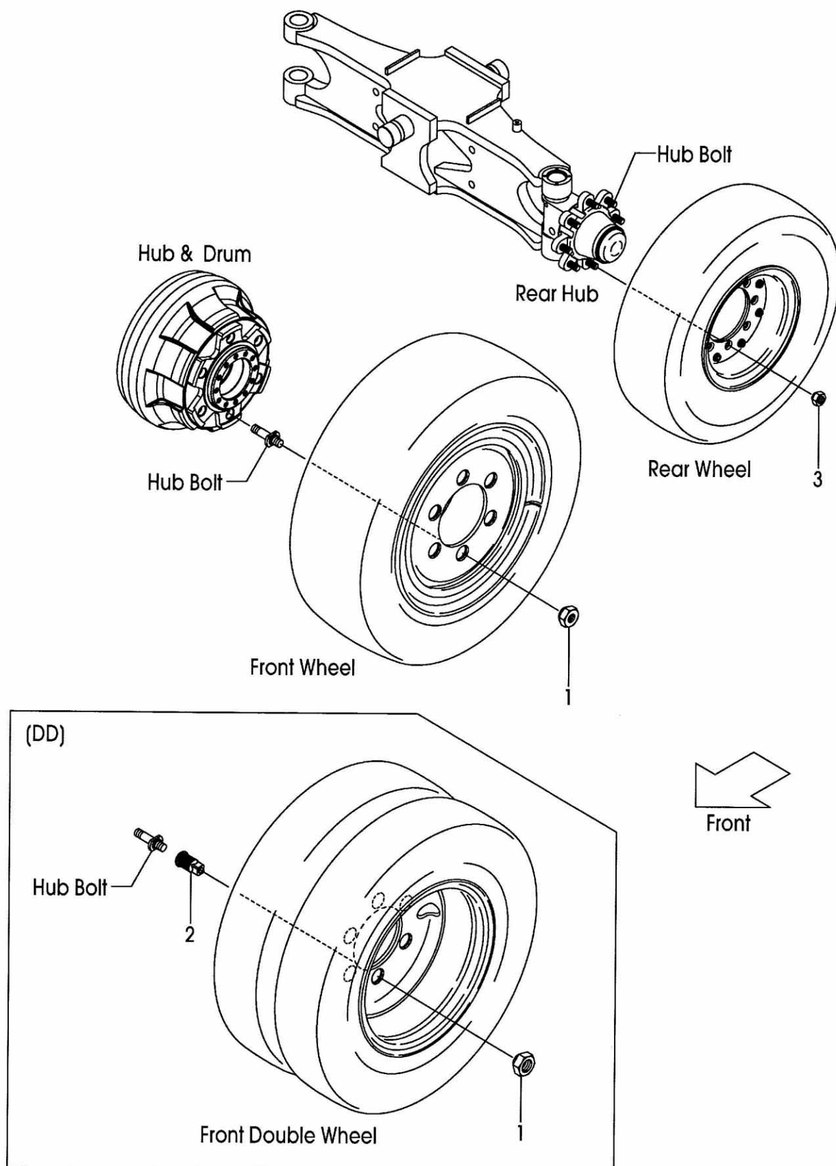
FIG.77 HUB NUT (F7C34410) ハブナット
