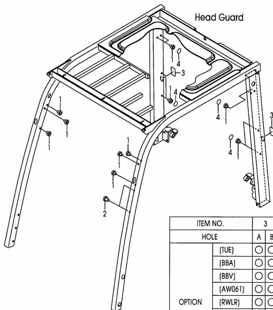
FIG.101 POP RIVET [TUE][BBA][BBV][AW061][RWL][RRE][FE] (F7C351C0) ホップリベット
