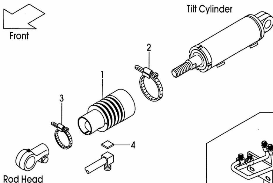
FIG.160 TILT BOOT [TLB] (F7C38520) ティルトブーツ
