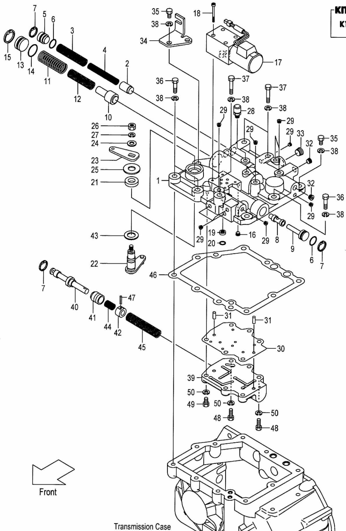
FIG.59 CONTROL VALVE (F7C325C0) コントロールバルブ
