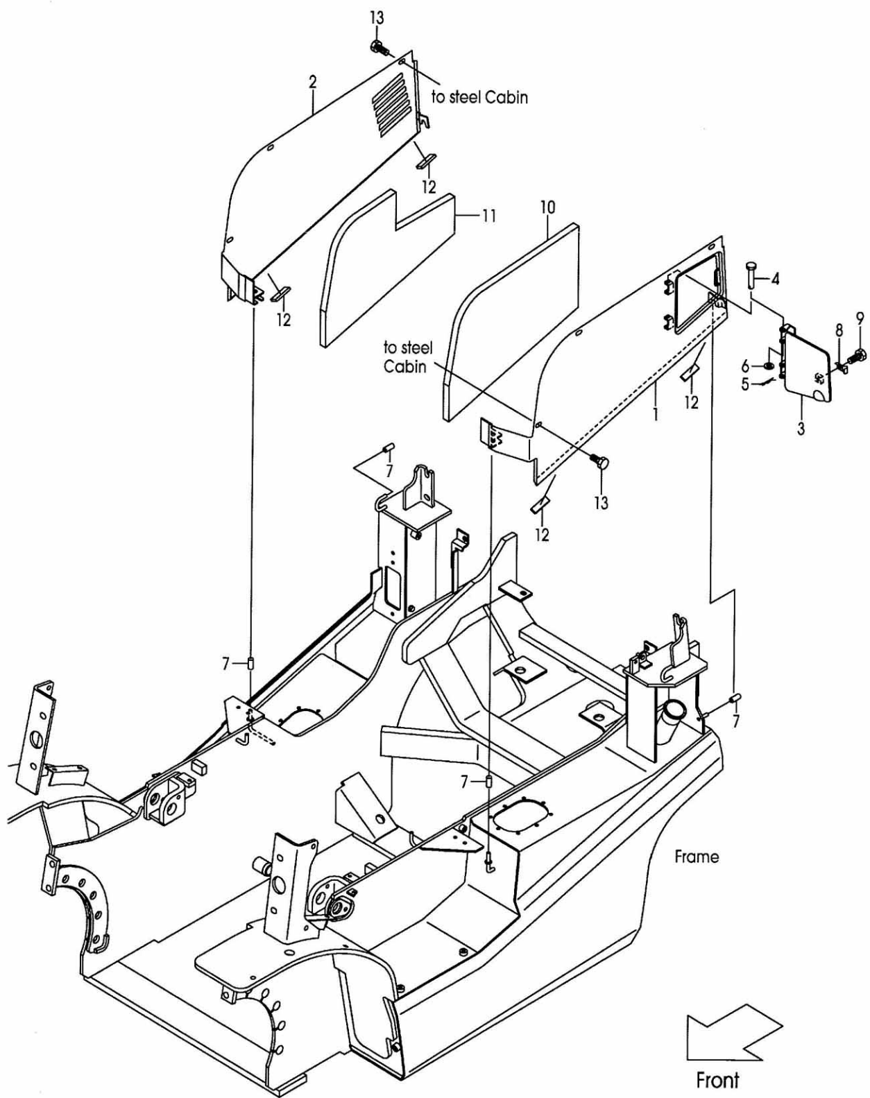
FIG.127 SIDE COVER [SCB001][SCBCR] (F7C364B0) サイドカバー
