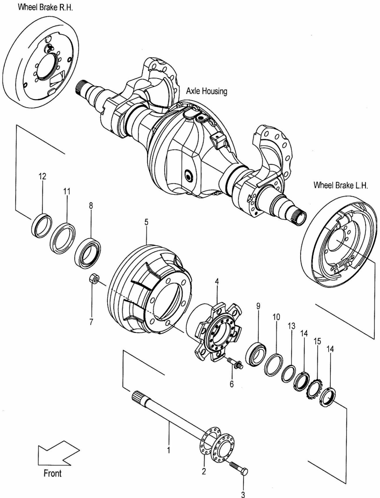
FIG.61 DRUM HUB (F7C33020) ドラムハブ
