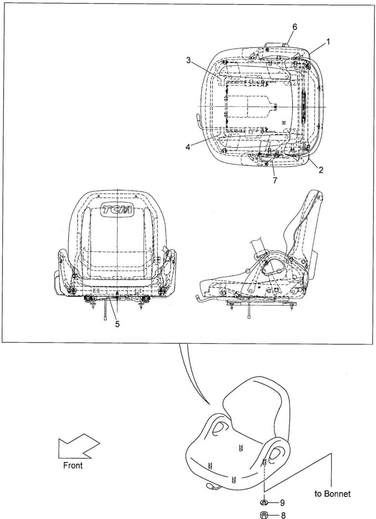
FIG.130 SEAT [HGL] (F7C36820) シート
