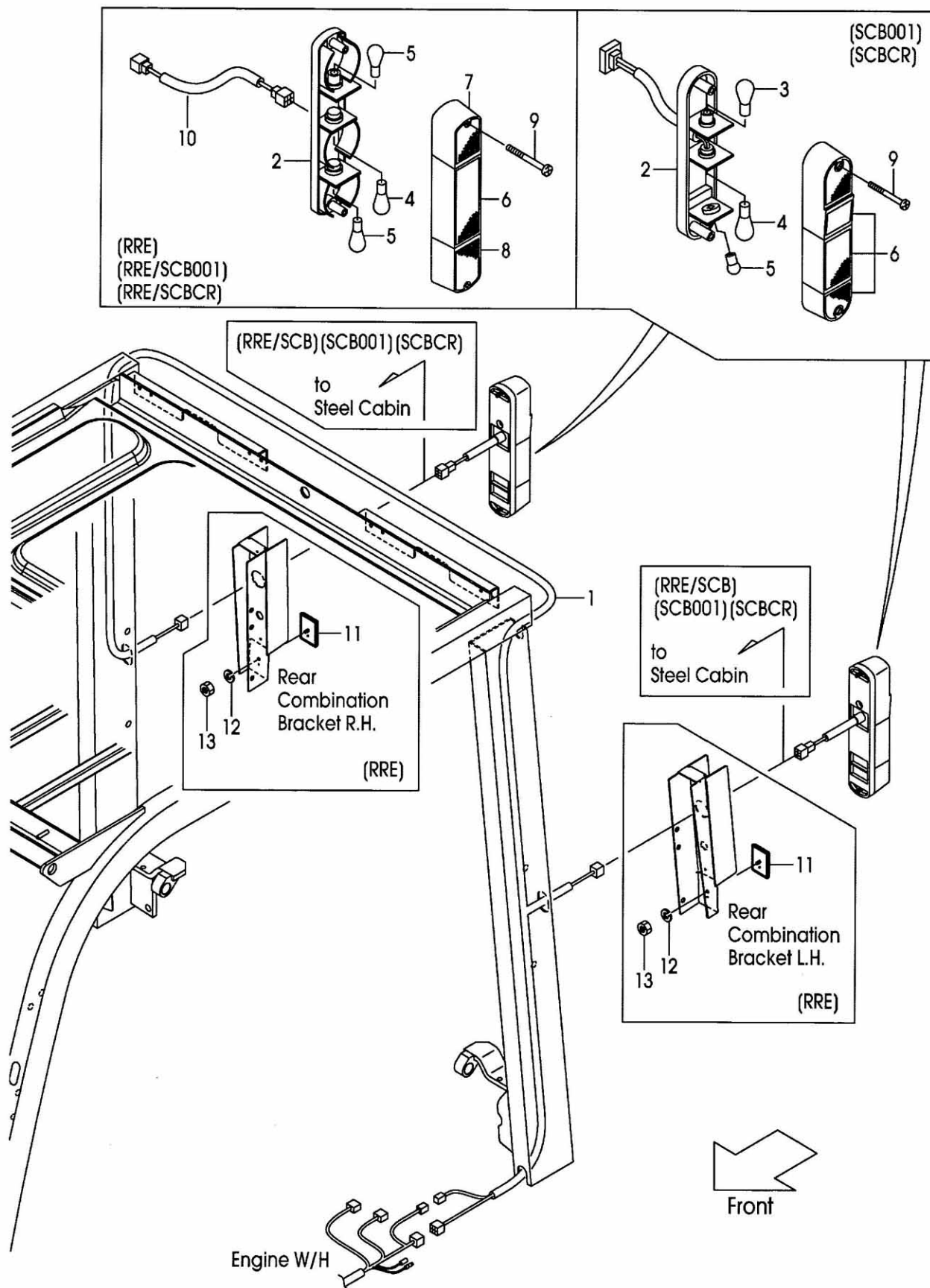
FIG.25 REAR COMBINATION LAMP [RRE][SCB001][SCBCR] (F7C324J0) リヤコンビネーションランプ
