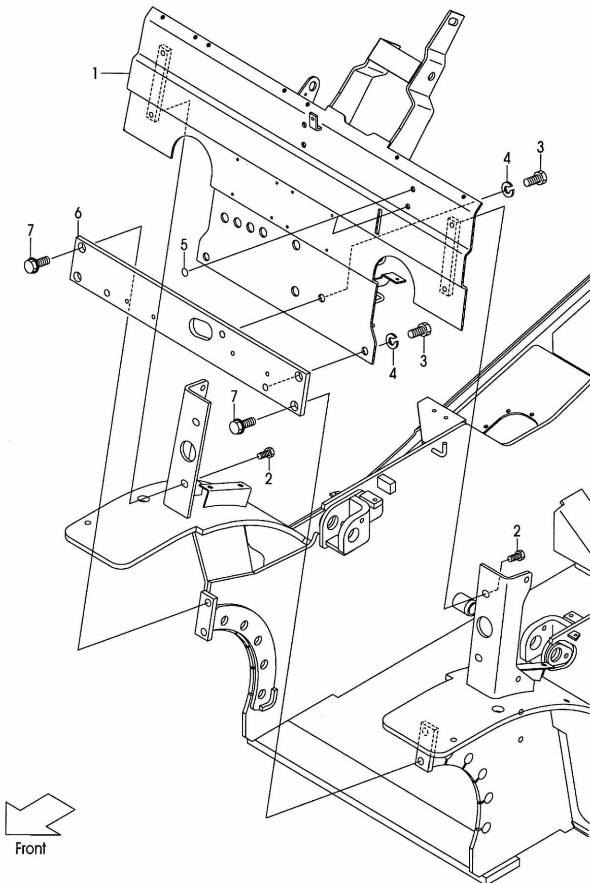
FIG.118 FRONT GUARD (F7C36410) フロントガード
