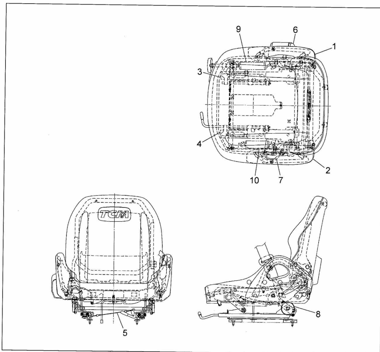
FIG.129 SEAT (F7C36810) シート
