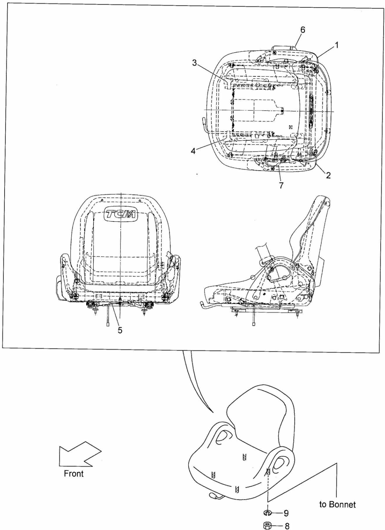
FIG.135 SEAT [EXB/HGL][EXC/HGL][EXK/HGL] (F7C36890) シート
