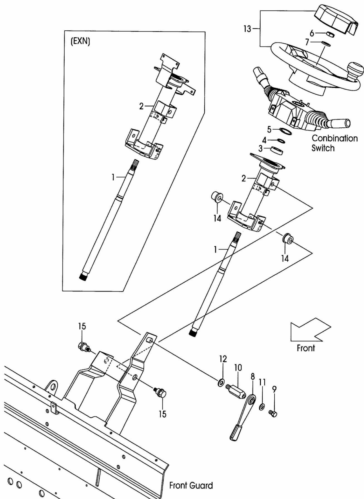
FIG.67 STEERING WHEEL UNIT (F7C34110) ステアリングホイールユニット
