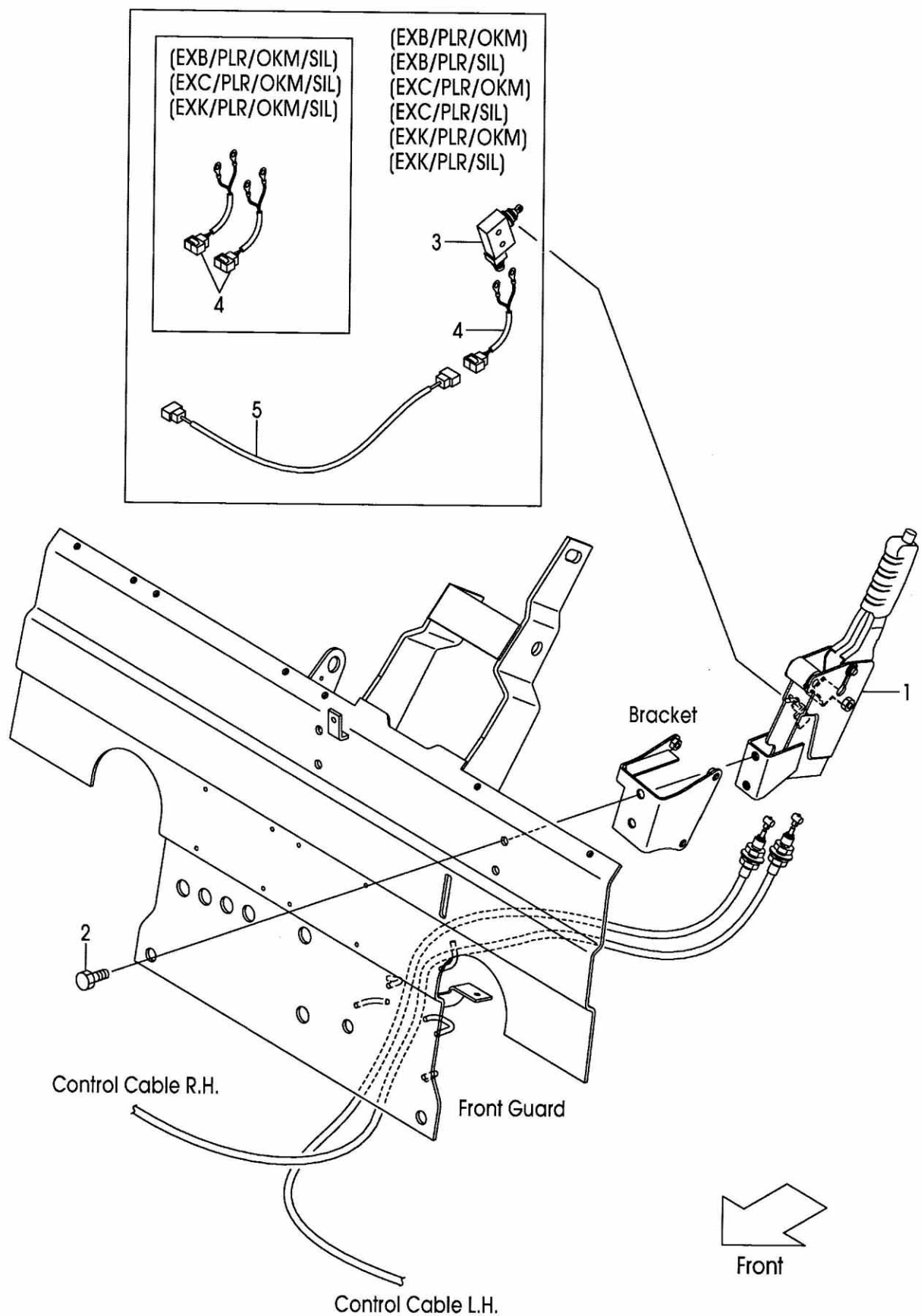
FIG.111 BRAKE LEVER [EXB/PLR][EXC/PLR][EXK/PLR] (F7C35540) ブレーキレバー
