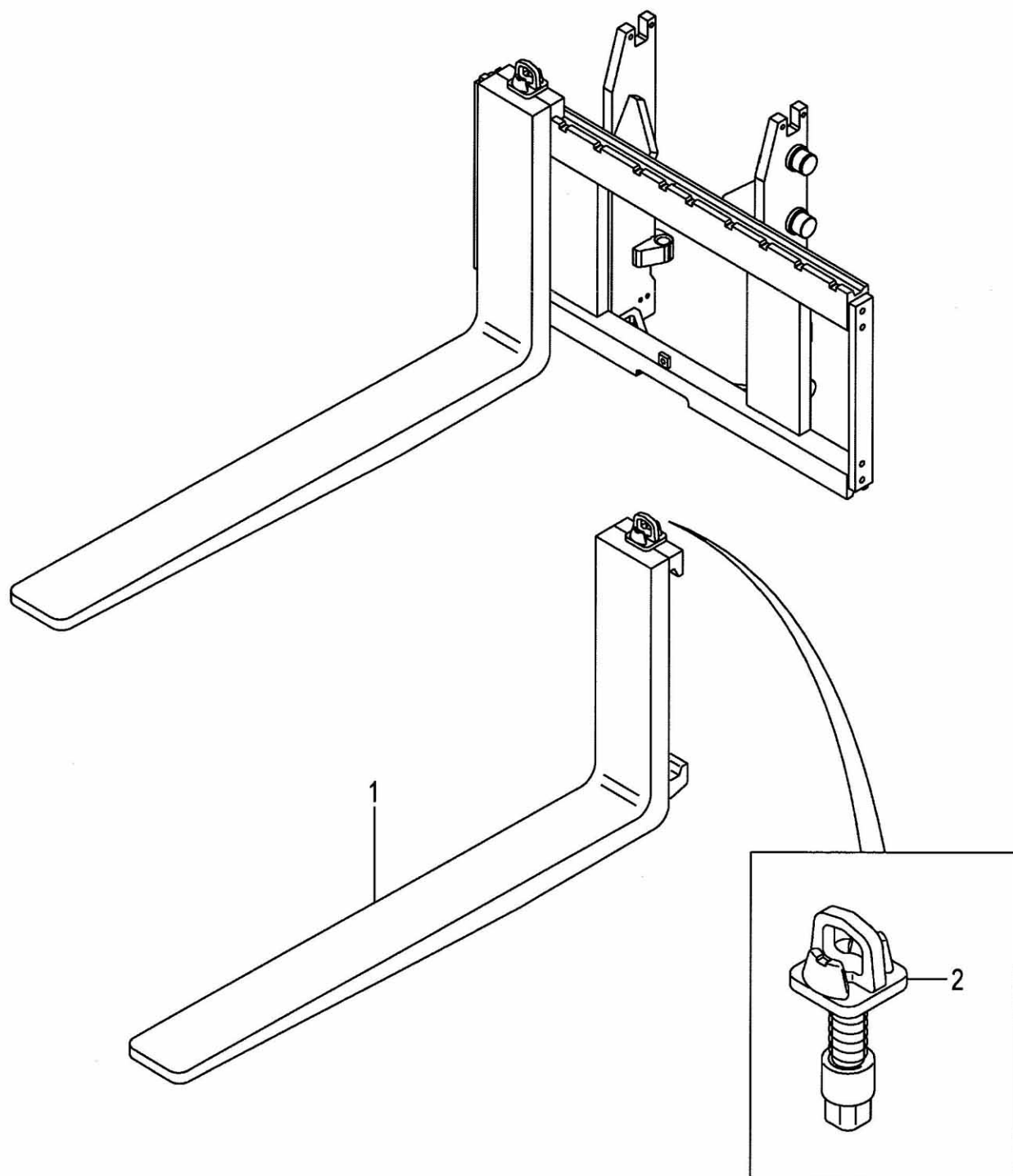
FIG.180 FORK [VM2Y5] (M7038110) フォーク
