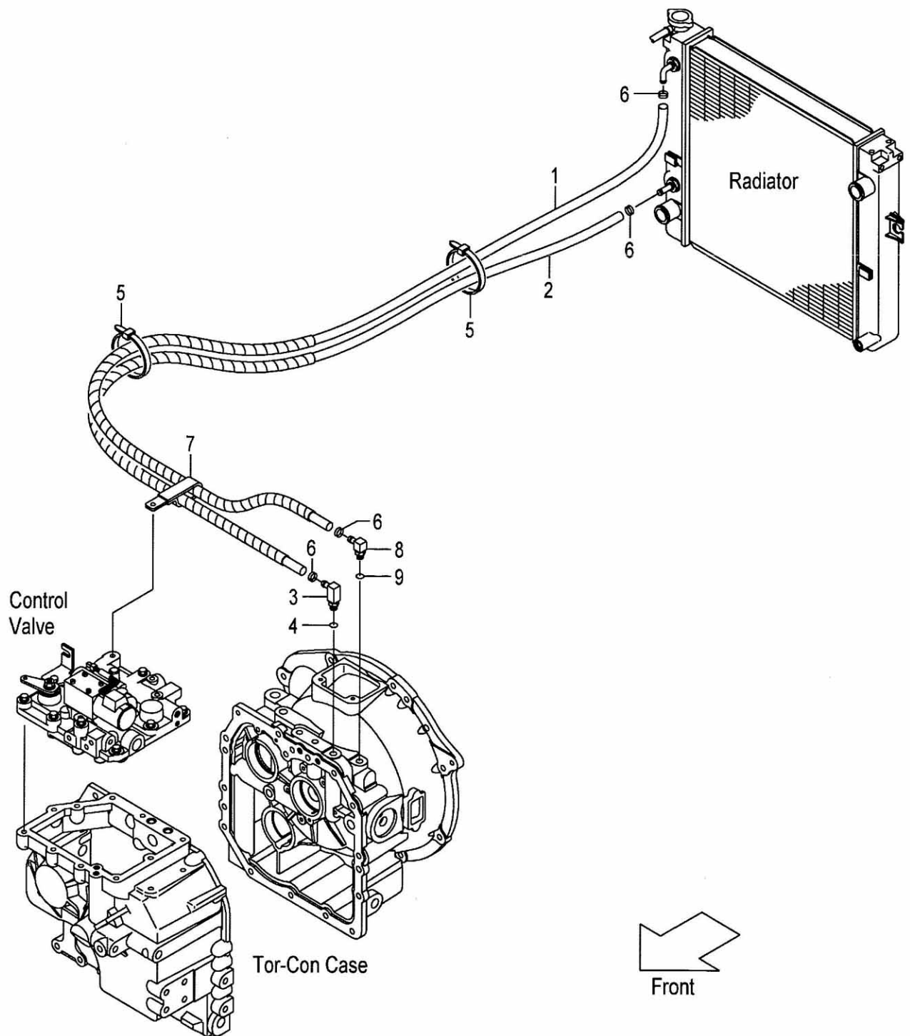
FIG.158 HYDRAULIC LINE (TOR-CON) (F7C376B0) ハイドロリックライン(トルコン)
