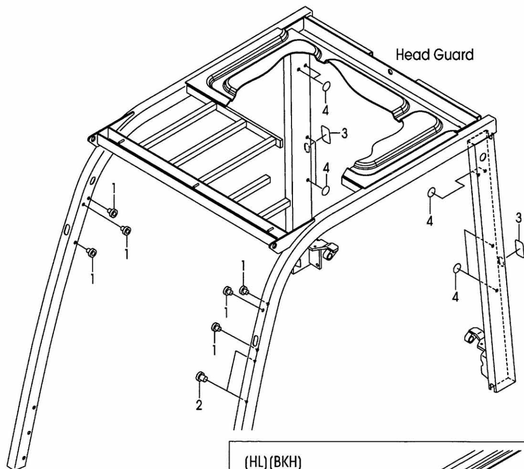
FIG.100 POP RIVET (F7C351B0) ホップリベット
