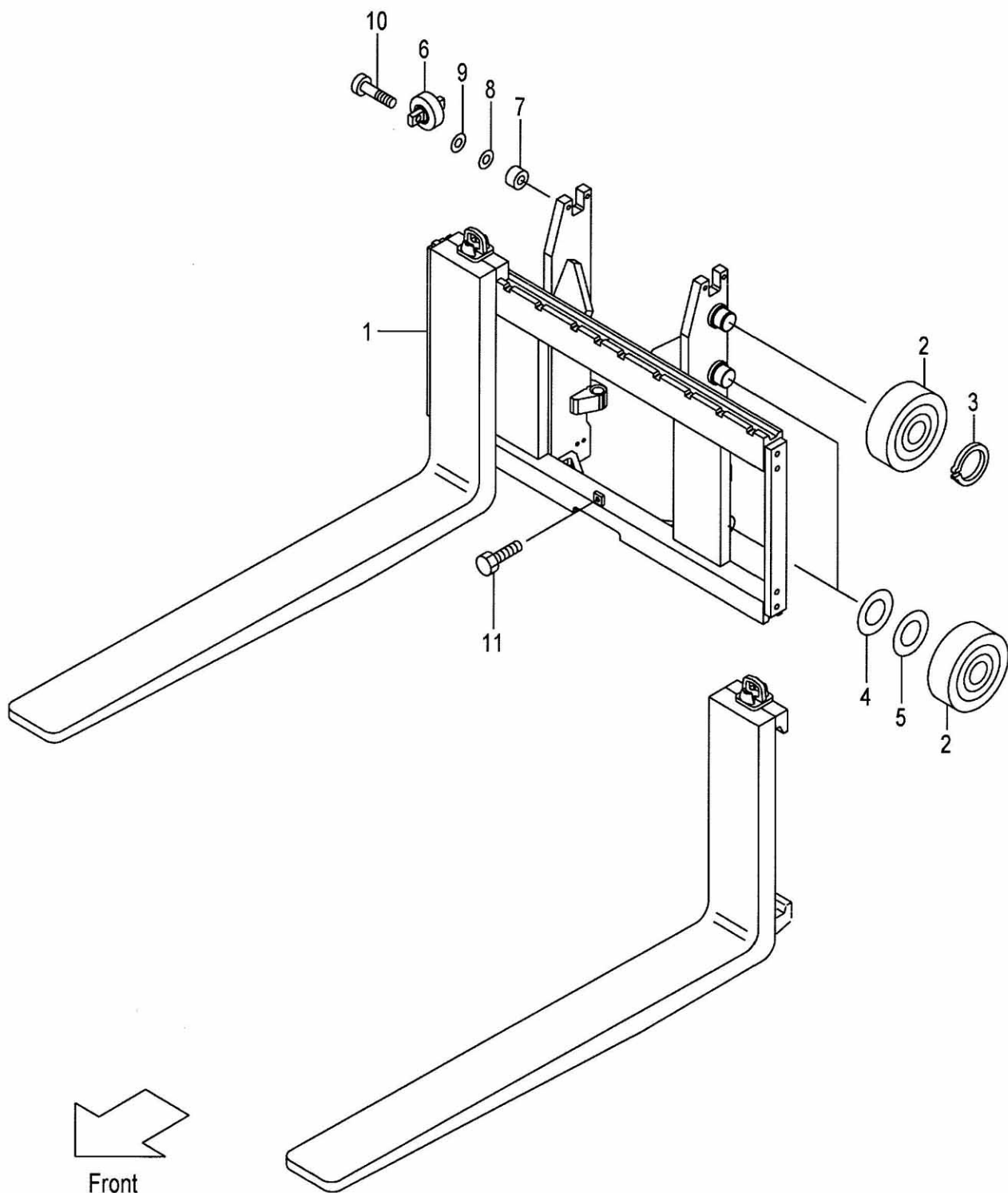
FIG.181 LIFT BRACKET [VM2Y5] (M7038210) リフトブラケット
