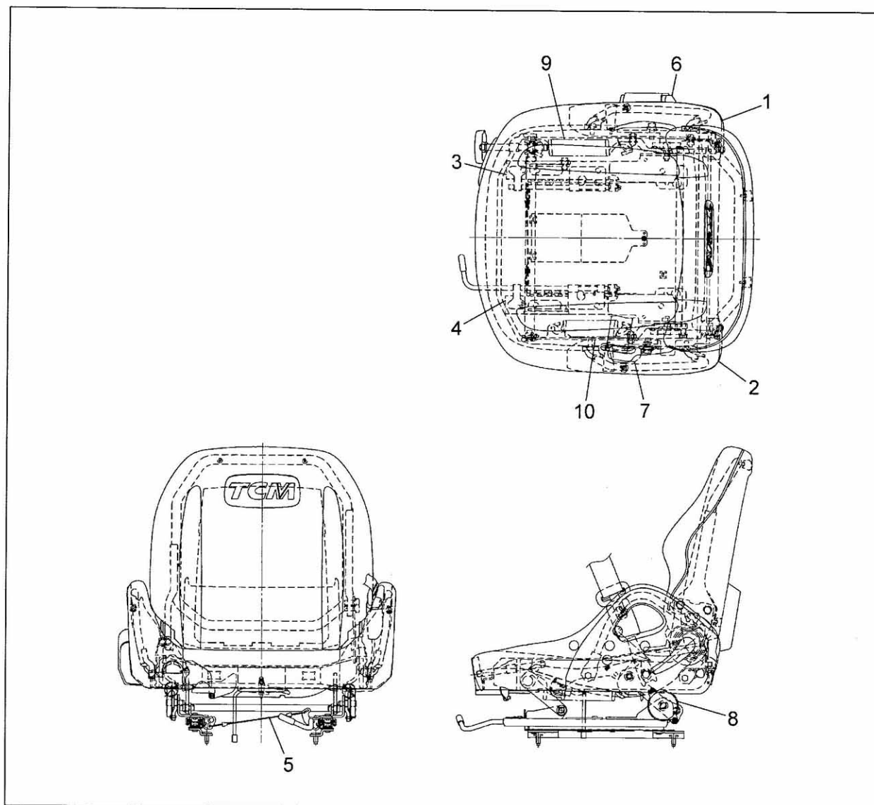
FIG.134 SEAT [EXB][EXC][EXK] (F7C36880) シート
