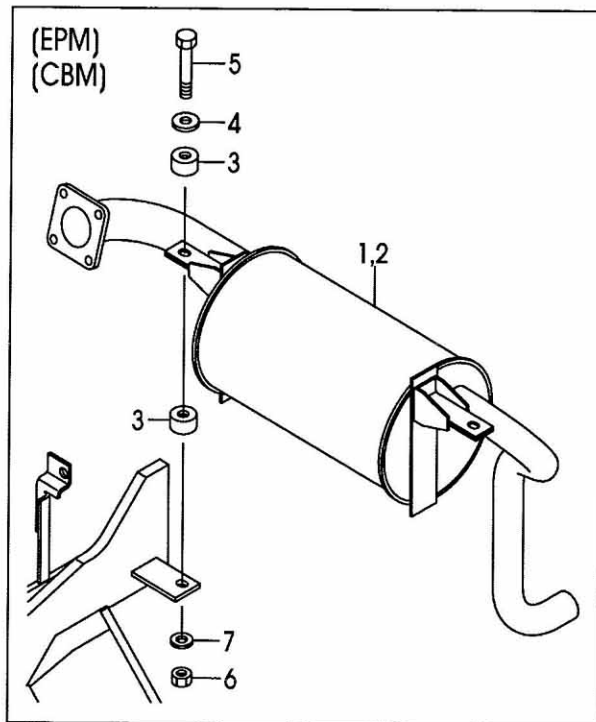
FIG.11 EXHAUST SYSTEM (F7C32320) エキゾーストシステム
