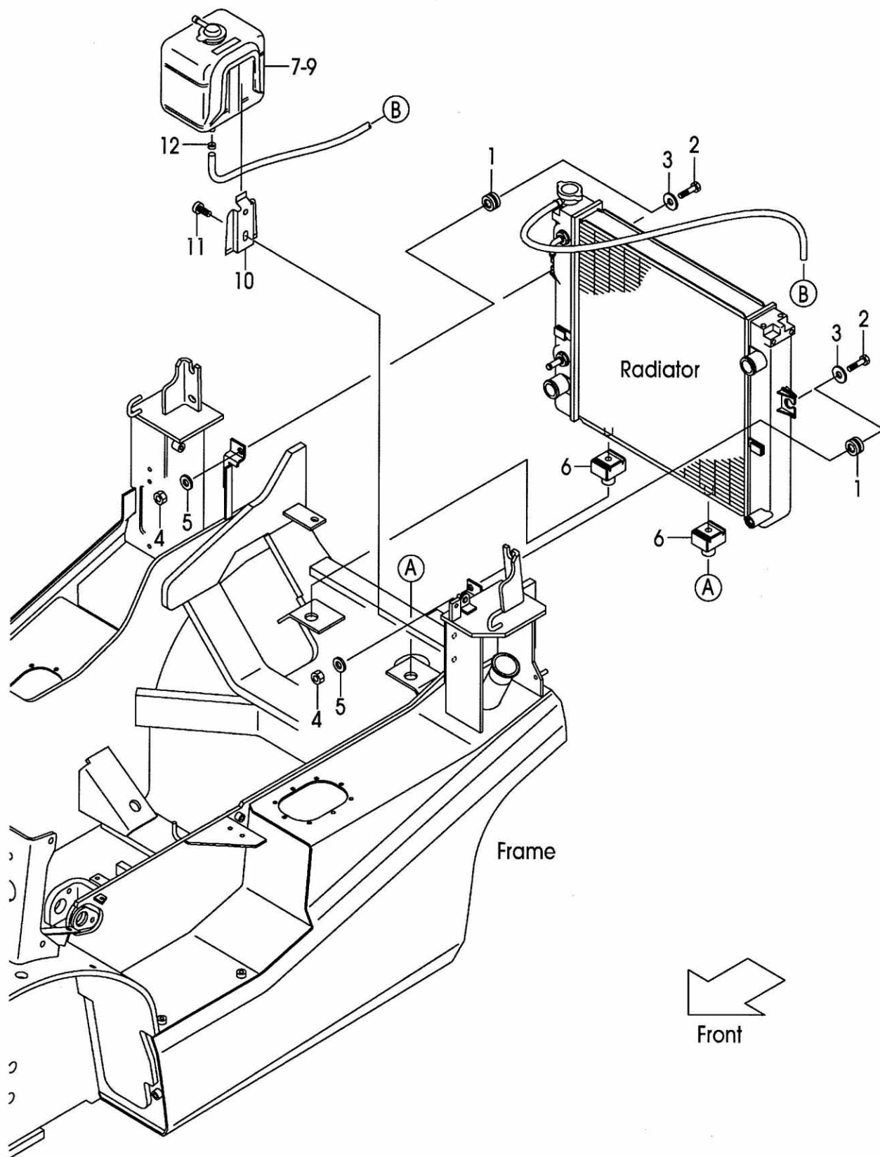
FIG.7 RADIATOR PARTS & RESERVE TANK (F7C32150) ラジエーターパーツ&リザーブタンク
