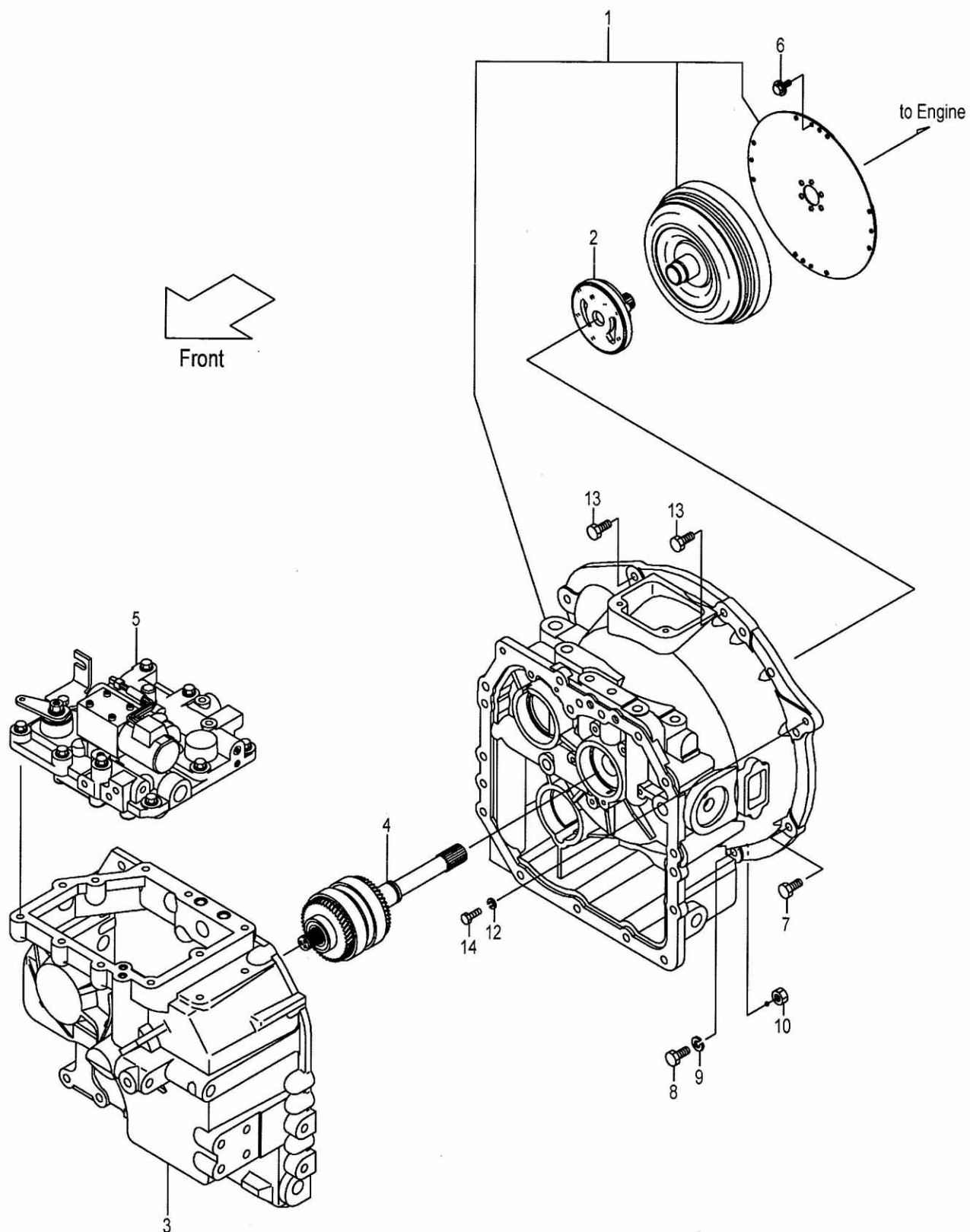
FIG.54 DRIVE UNIT MOUNT (F7C32520) ドライブユニットマウント
