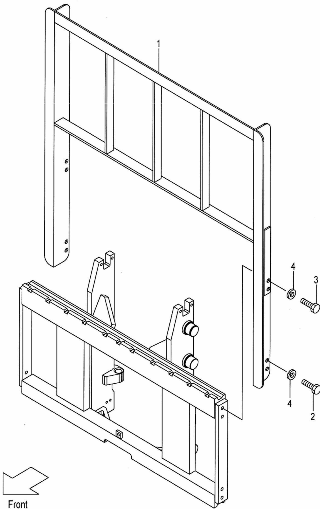
FIG.182 BACKREST [VM2Y5] (M7038220) バックレスト
