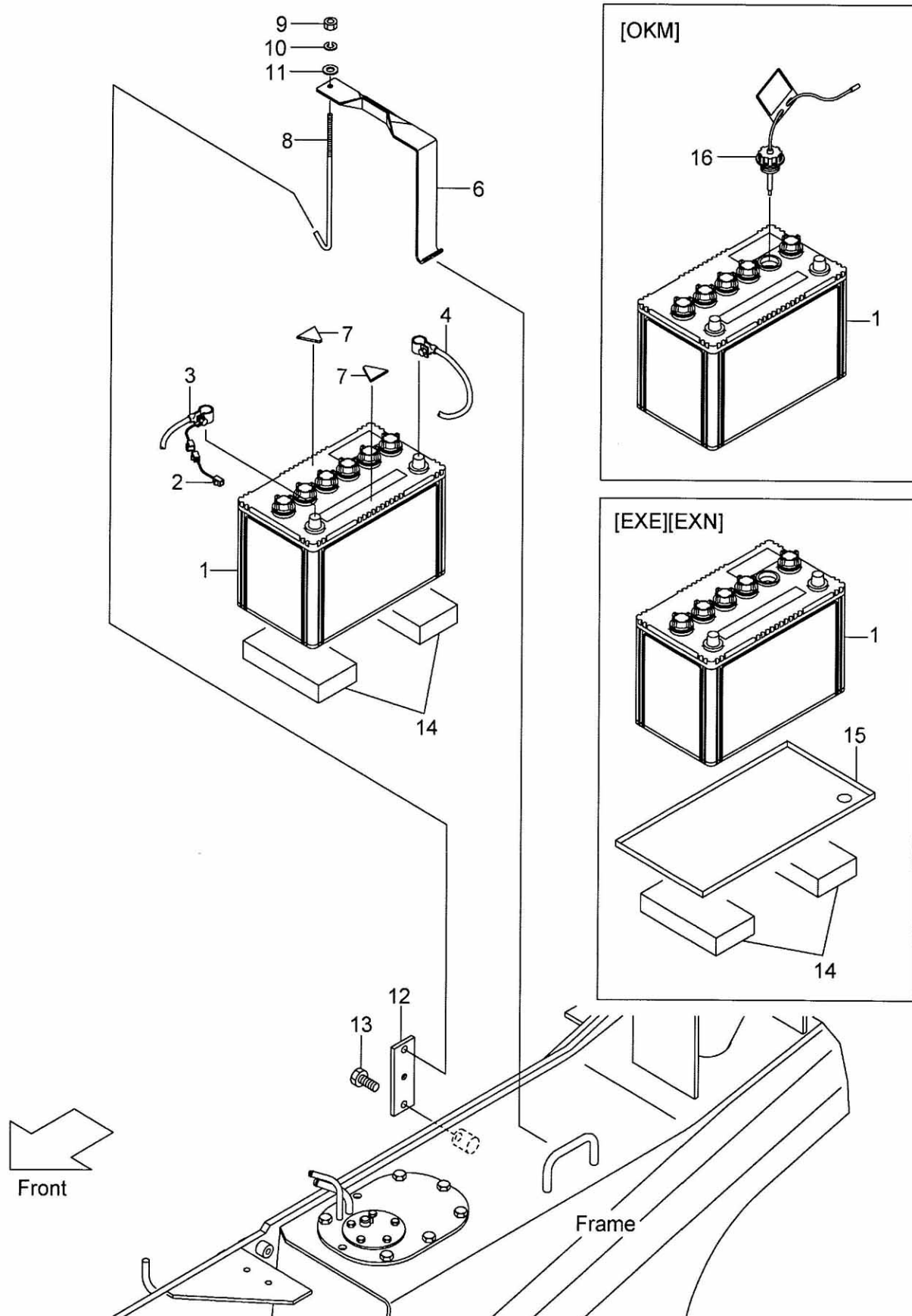
FIG.22 BATTERY (F7C324F0) バッテリー
