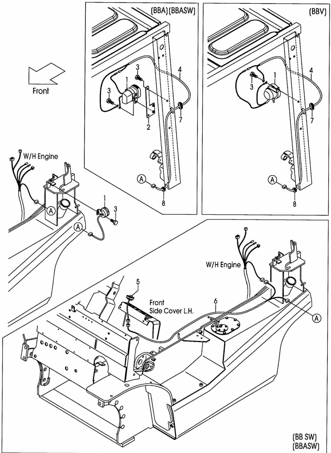
FIG.38 BACK BUZZER (F7C324X0) バックブザー
