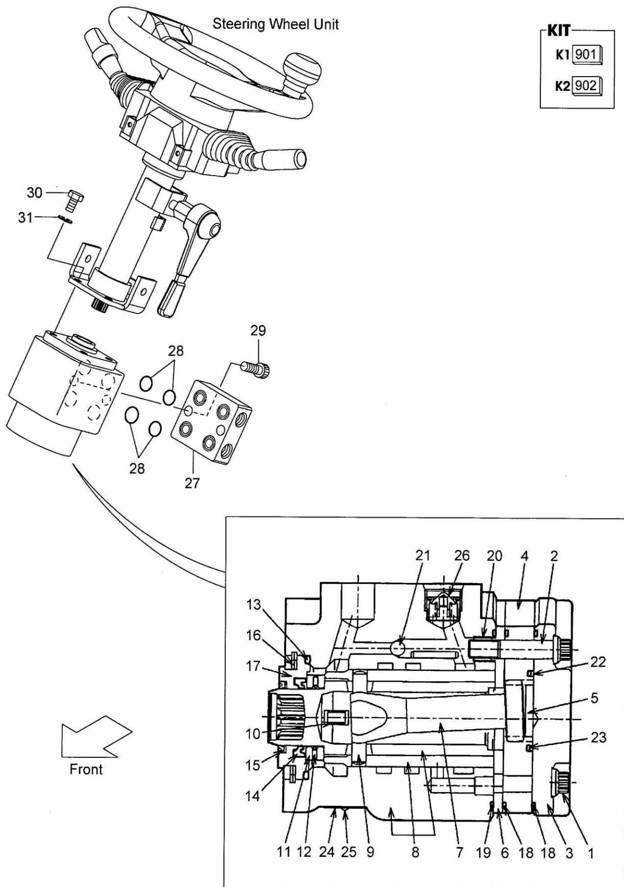
FIG.70 ORBITROL [EXE][EXK][EXN] (F7C34140) オービットロール
