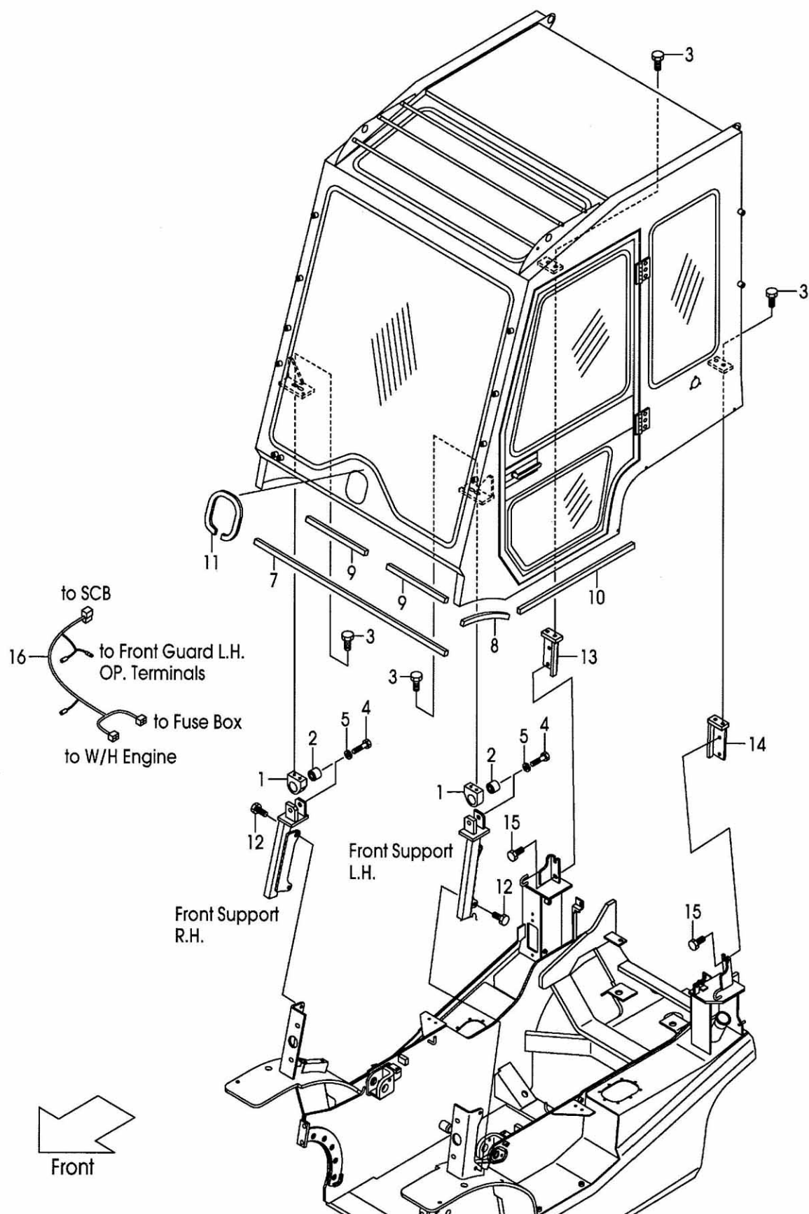
FIG.178 STEEL CABIN MOUNT [SCB001][SCBCR] (F7C393Q0) スチールキャビンマウント
