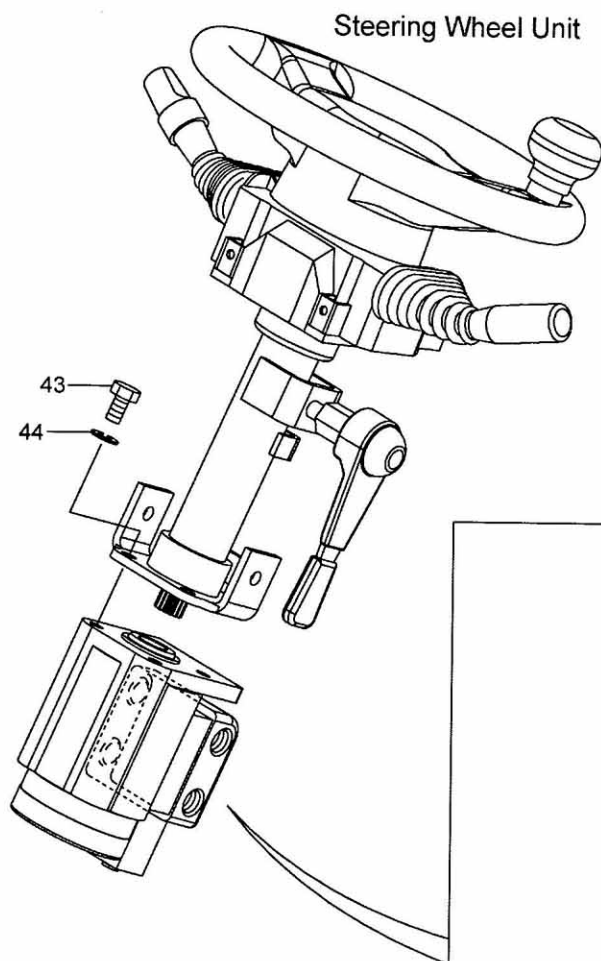
FIG.69 ORBITROL (F7C34130) オービットロール
