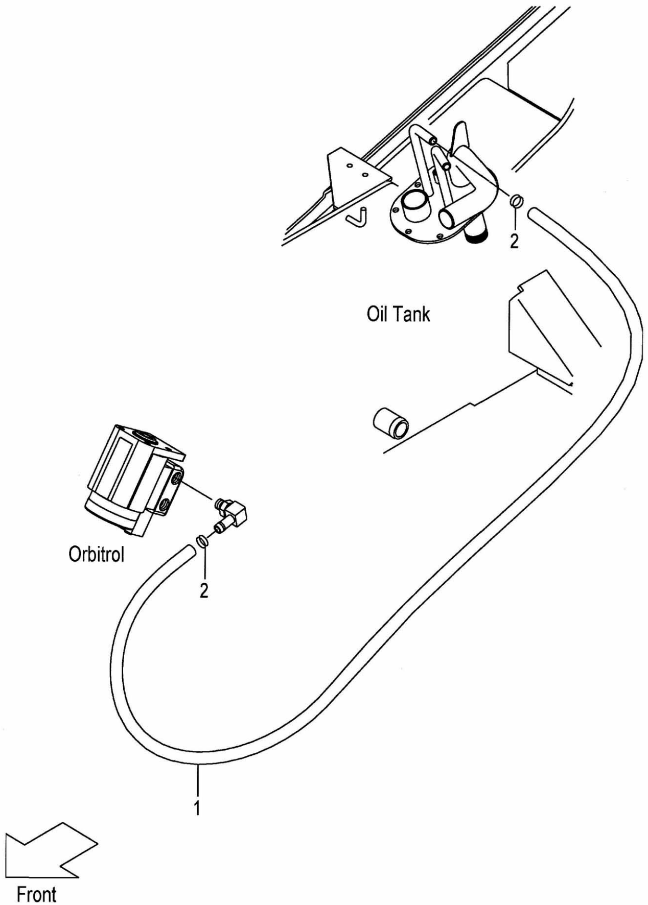
FIG.156 HYDRAULIC LINE (MAIN)(3/4) (F7C37660) ハイドロリックライン(メイン)(3/4)
