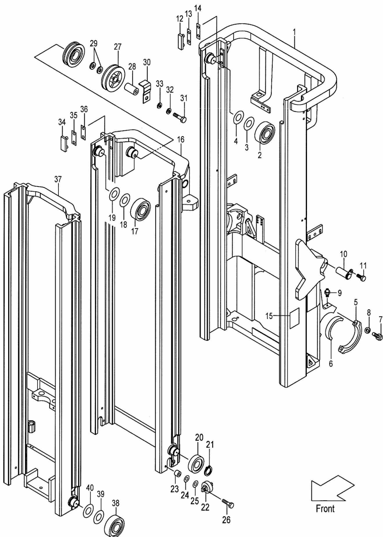
FIG.196 MAST [VFHM2Y5] (M7030710) マスト
