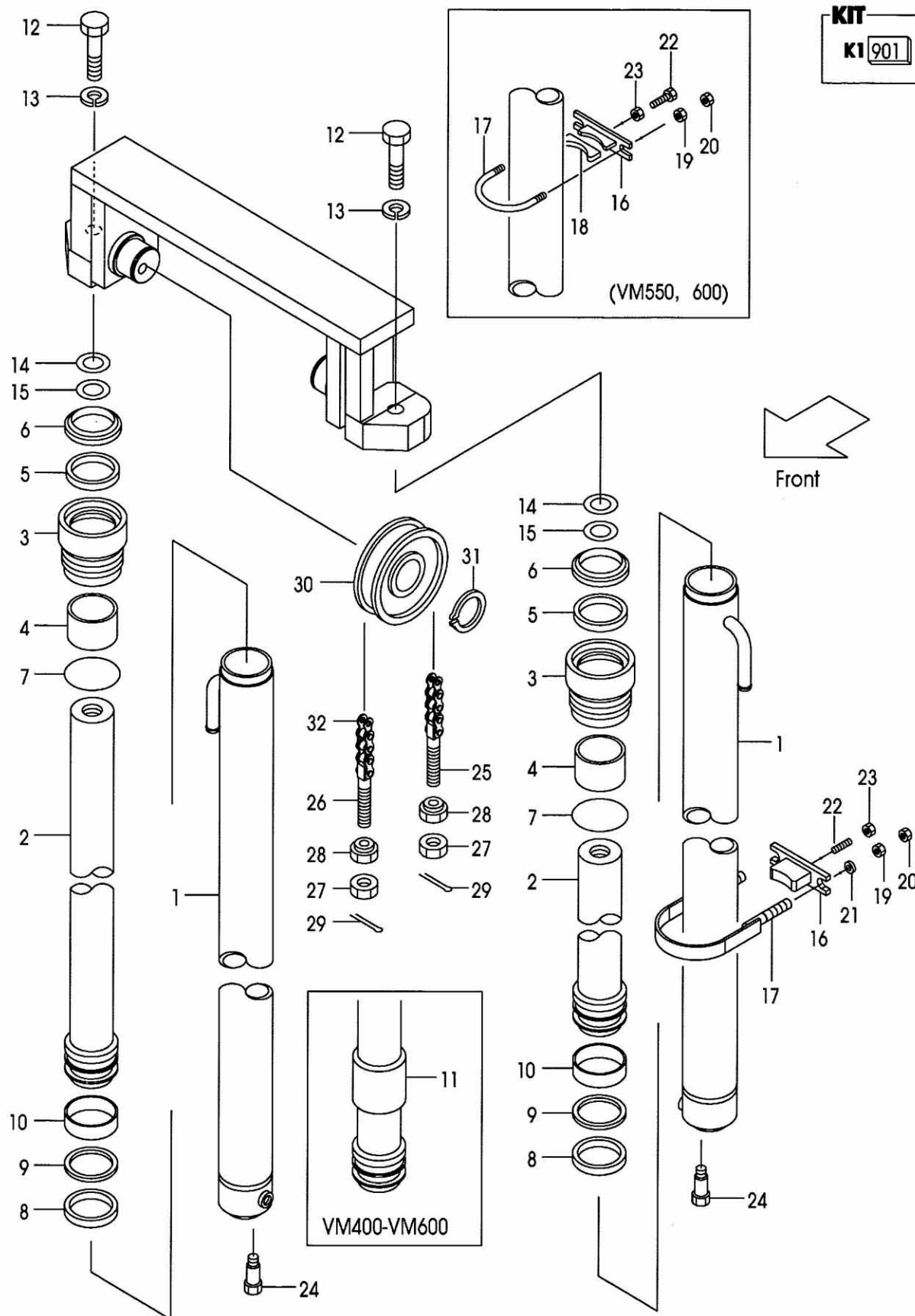
FIG.184 LIFT CYLINDER [VM2Y5] (M7038410) リフトシリンダ
