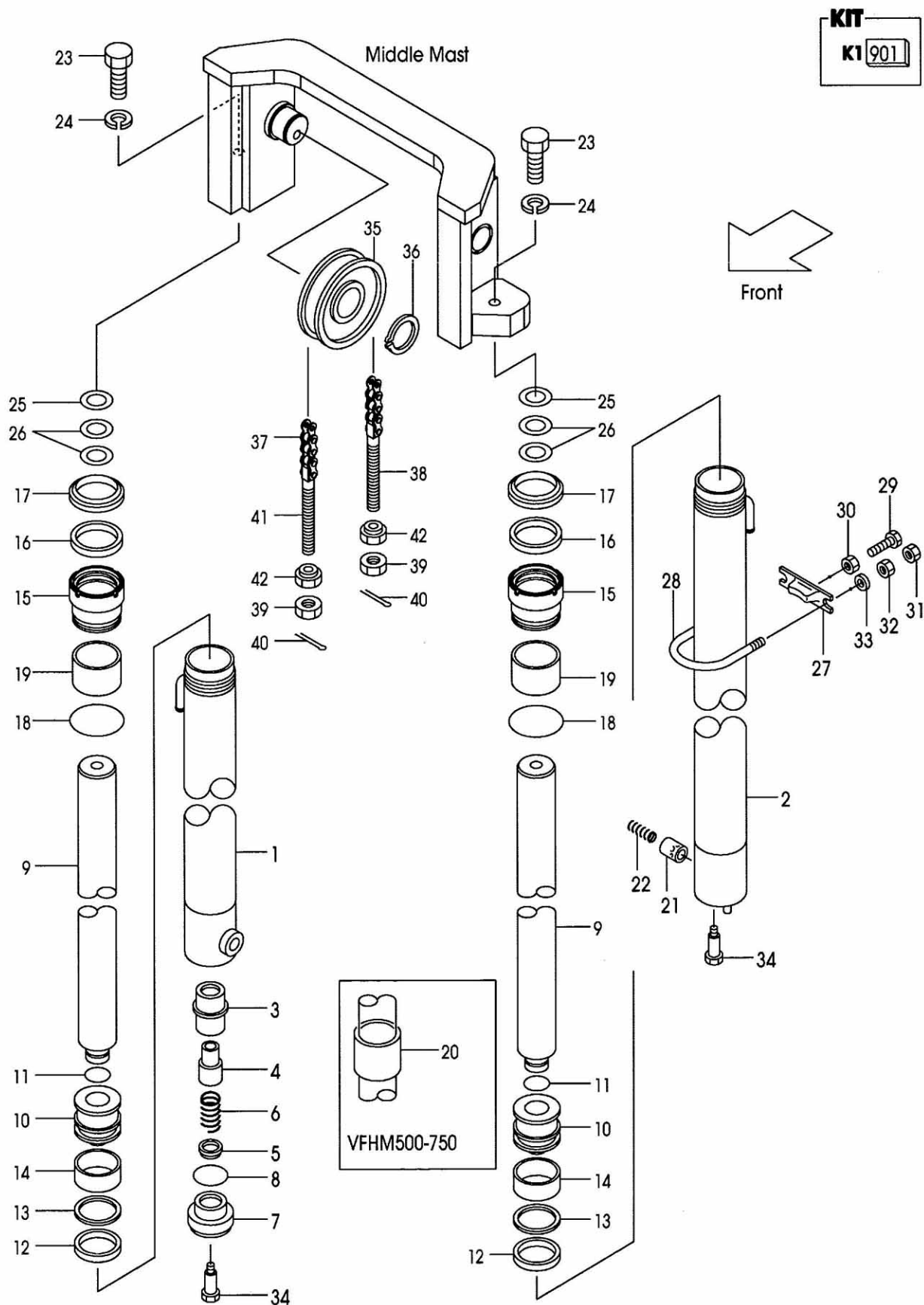
FIG.198 LIFT CYLINDER(REAR) [VFHM2Y5] (M7030820) リフトシリンダ(リヤ)
