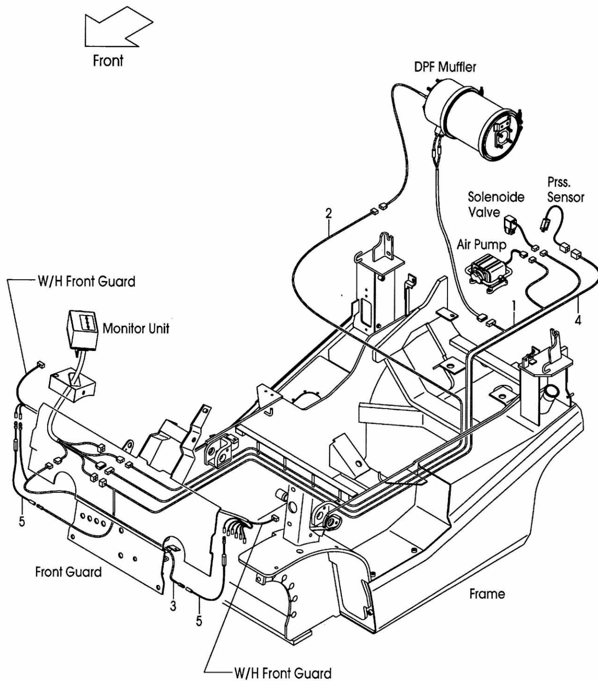
FIG.14 DPF WIRE HARNESS [DPF] (F7C32360) DPFワイヤハーネス
