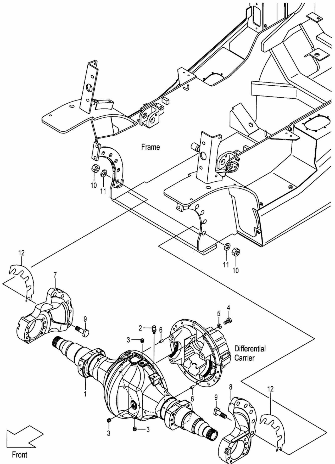
FIG.60 DRIVE AXLE (F7C33010) ドライブアクスル
