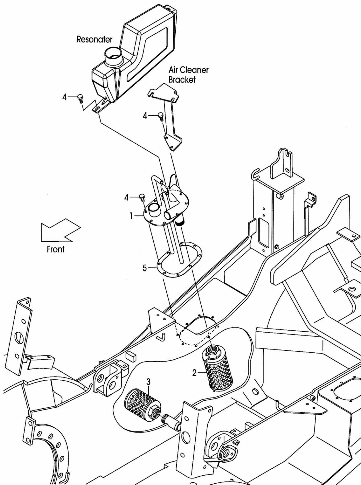
FIG.113 OIL TANK (F7C36120) オイルタンク
