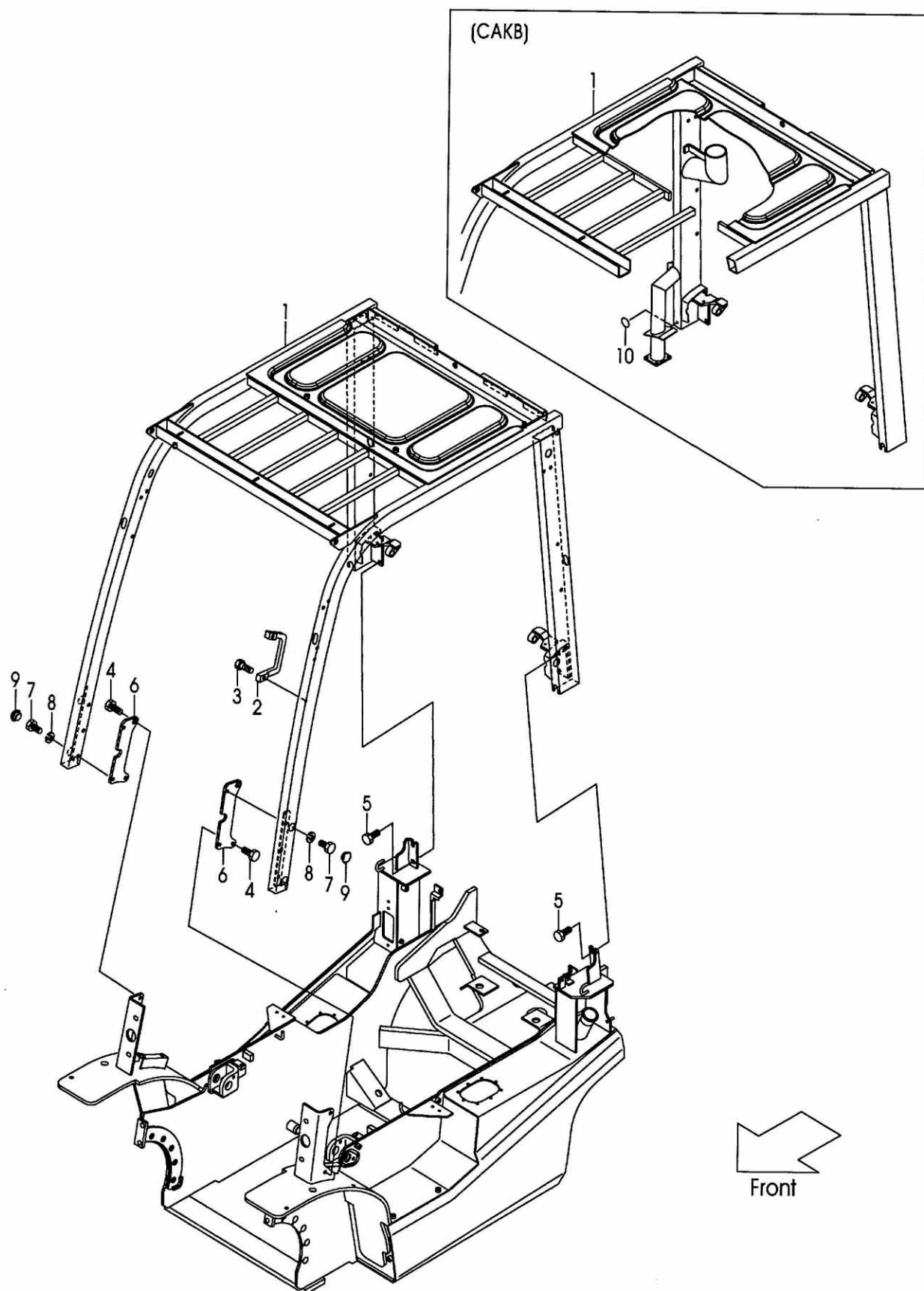
FIG.93 OVERHEAD GUARD (F7C35110) オーバヘッドガード
