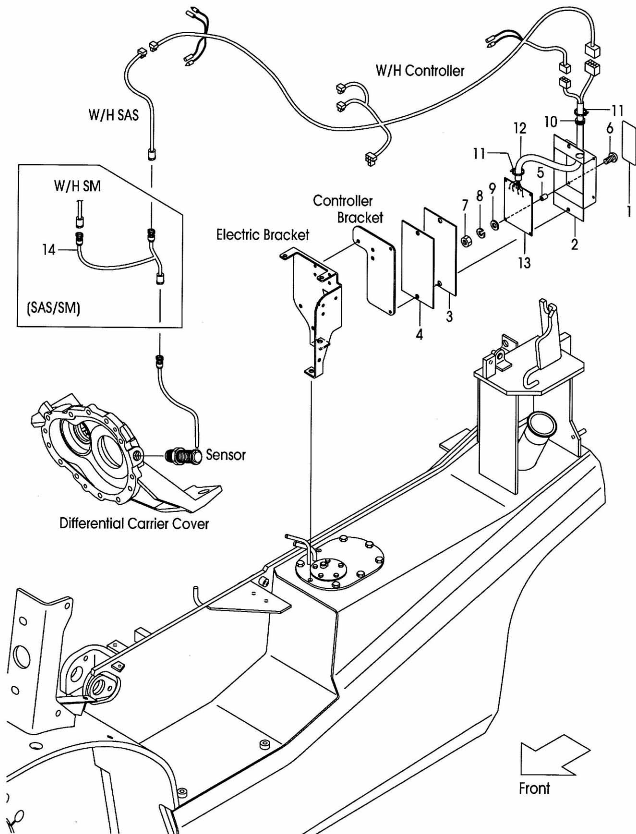
FIG.49 SPEED DETECTOR UNIT [SAS] (F7C326E0) スピードデテクタユニット
