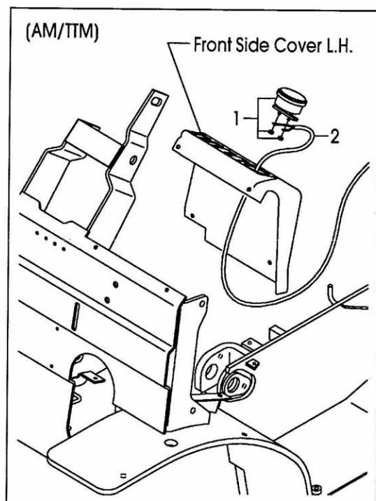
FIG.45 AMMETER [AM] (F7C326A0) アンメータ
