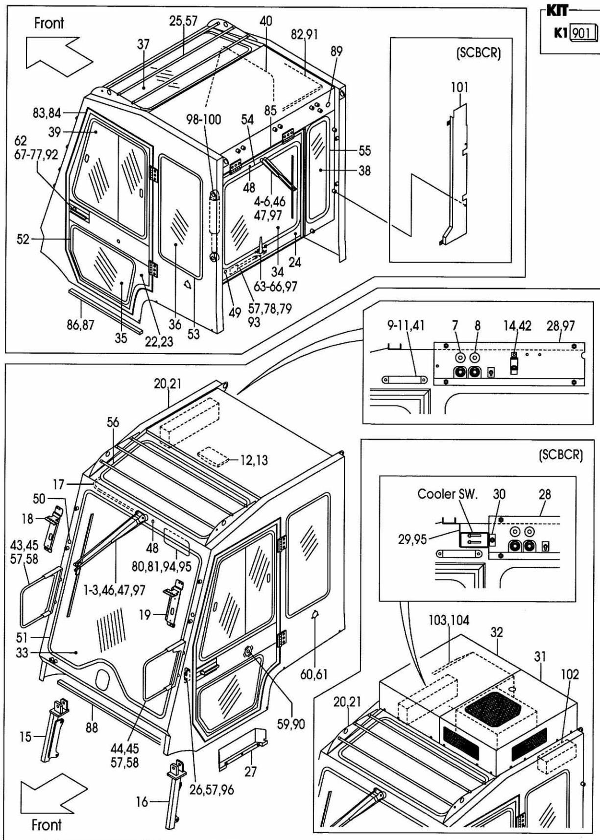
FIG.175 STEEL CABIN [SCB001][SCBCR] (F7C393M0) スチールキャビン
