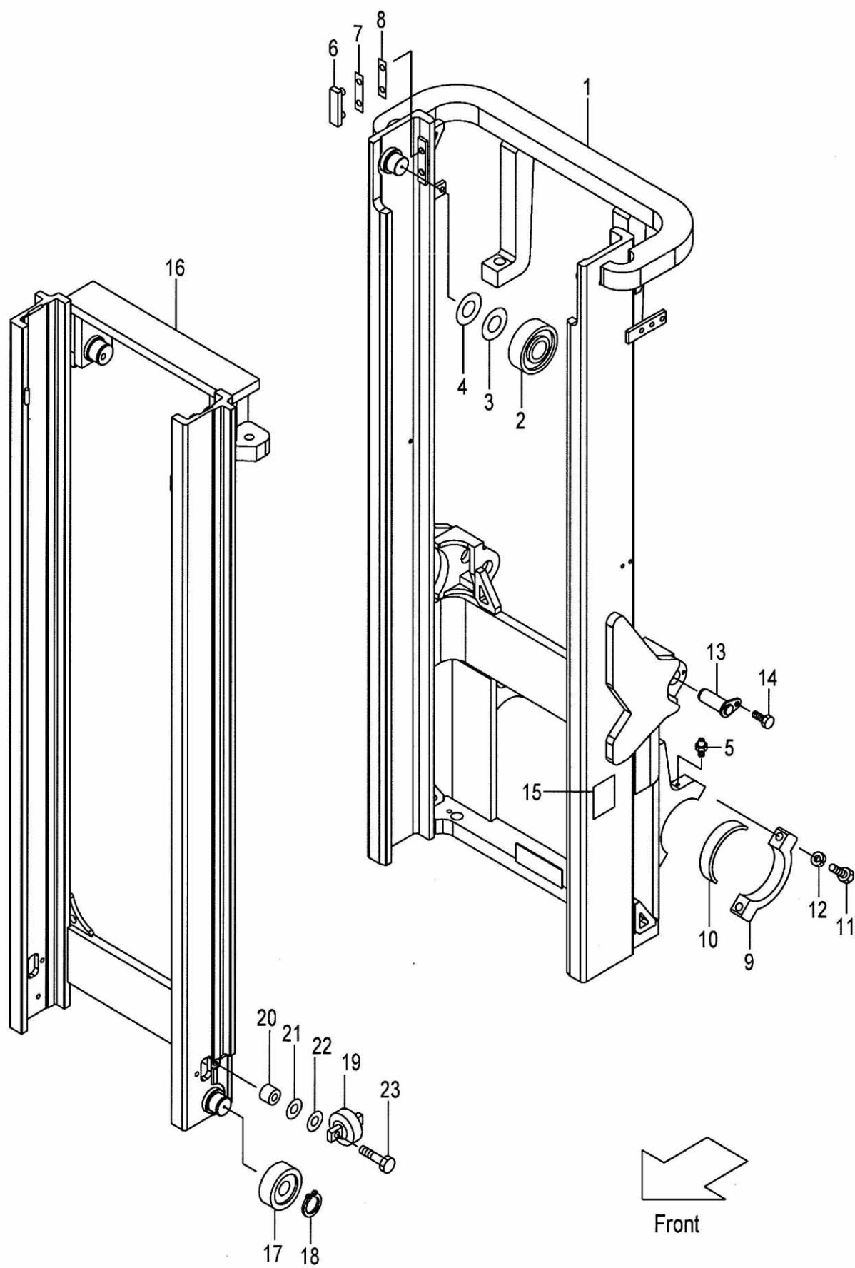
FIG.183 MAST [VM2Y5] (M7038310) マスト
