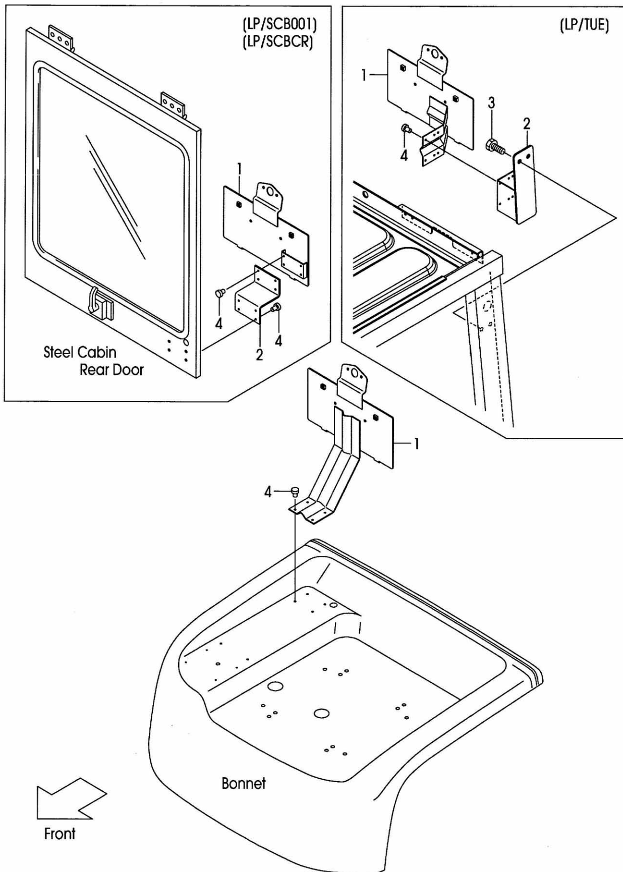
FIG.28 LICENSE LAMP [LP] (F7C324N0) ライセンスランプ
