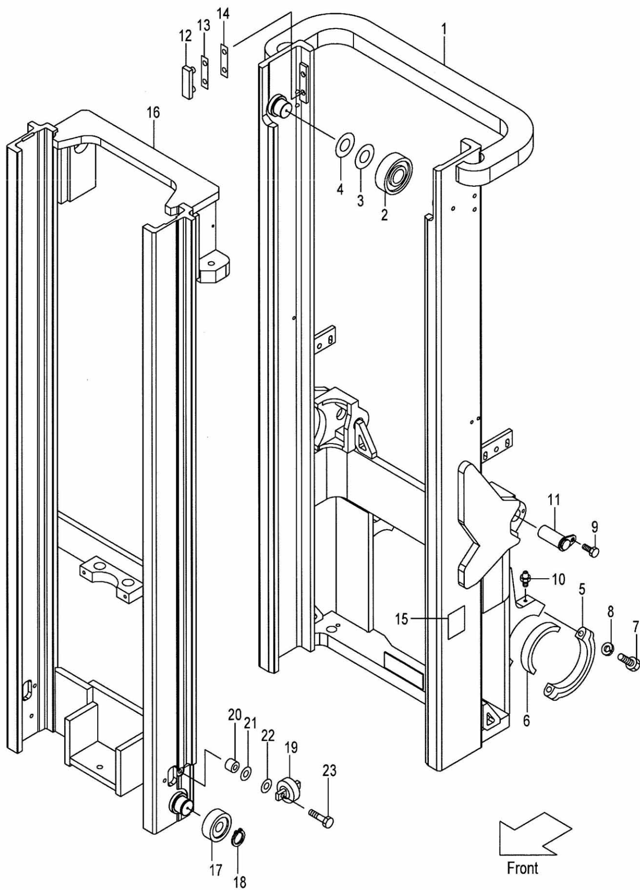
FIG.189 MAST [VFM2Y5] (M7030410) マスト
