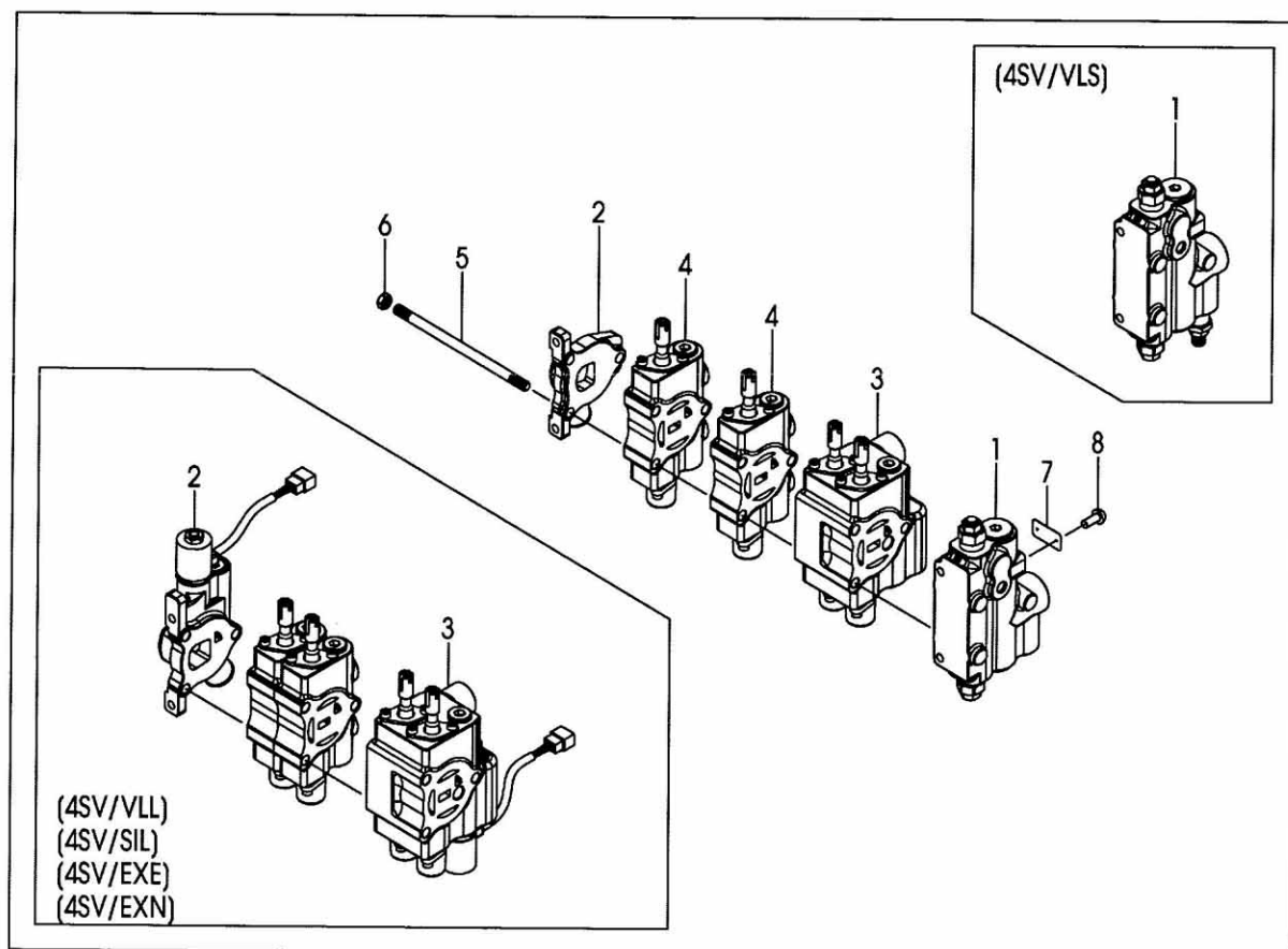
FIG.142 CONTROL VALVE [4SV] (F7C37330) コントロールバルブ
