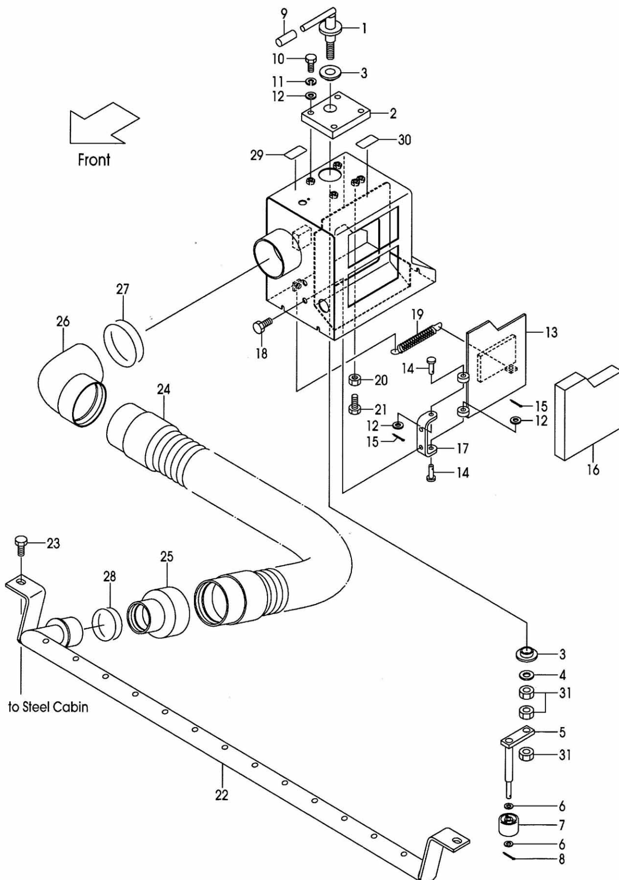
FIG.176 DEFROSTER [SCB001/DEF] (F7C393N0) デフロスター
