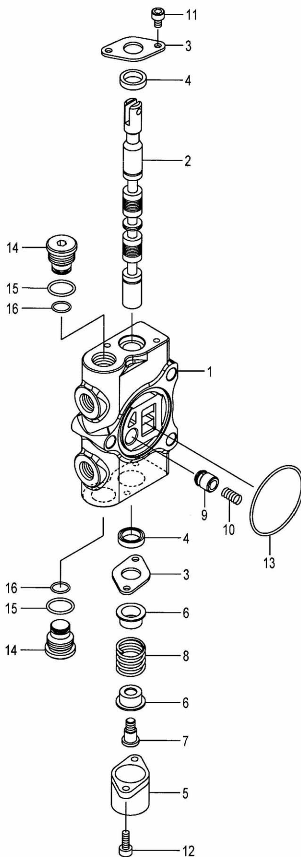
FIG.153 VALVE SECTION [3SV][4SV][5SV] (F7C373Q0) ハルブセクション
