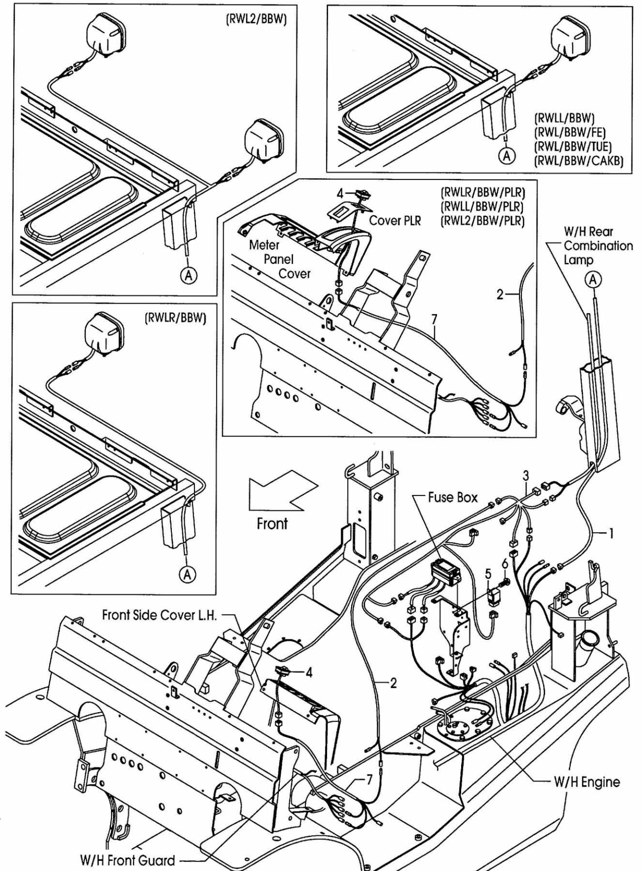
FIG.34 REAR WORKING LIGHT WIRE HARNESS [RWL/BBR] (F7C324U0) リヤワーキングライトワイヤハーネス
