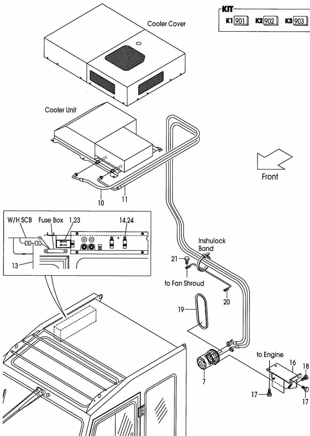
FIG.179 STEEL CABIN COOLER [SCBCR] (F7C393R0) スチールキャビンクーラー
