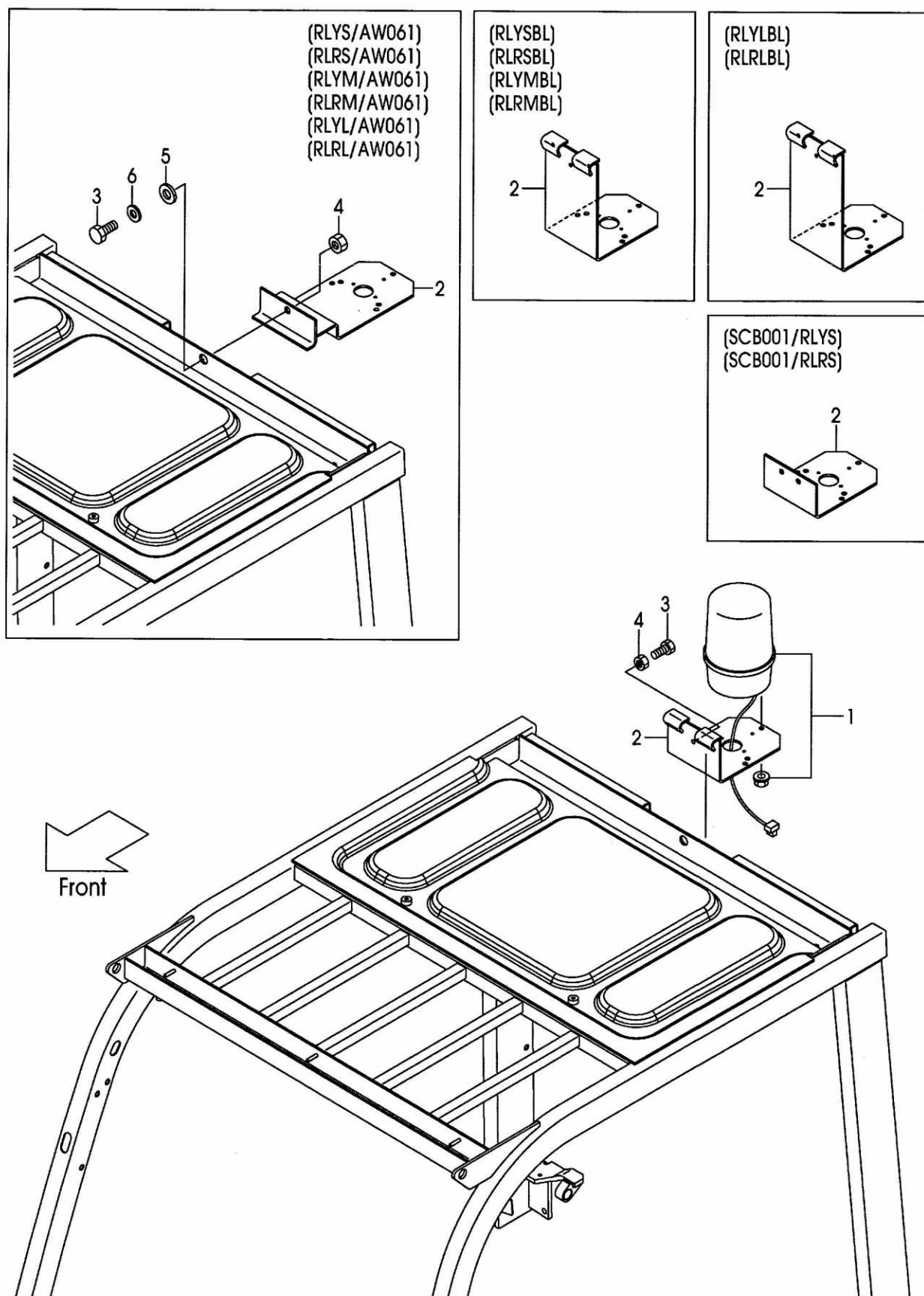
FIG.35 REVOLVING LIGHT [RLY][RLR] (F7C324V0) リボルビングライト
