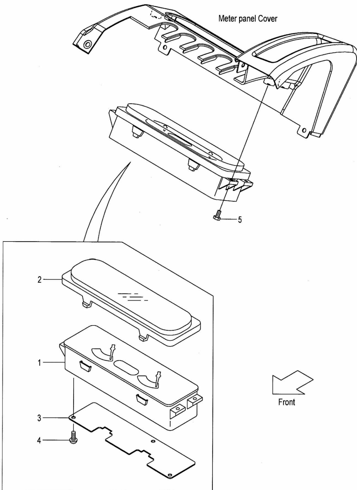
FIG.17 COMBINATION METER (F7C32410) コンビネーションメータ
