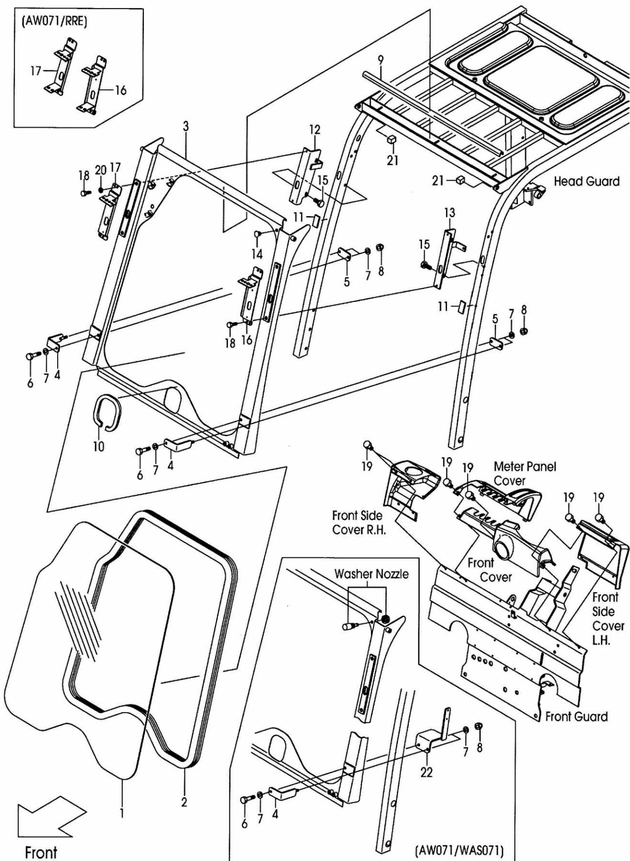
FIG.169 FRONT GLASS [AW061][AW071] (F7C39310) フロントガラス
