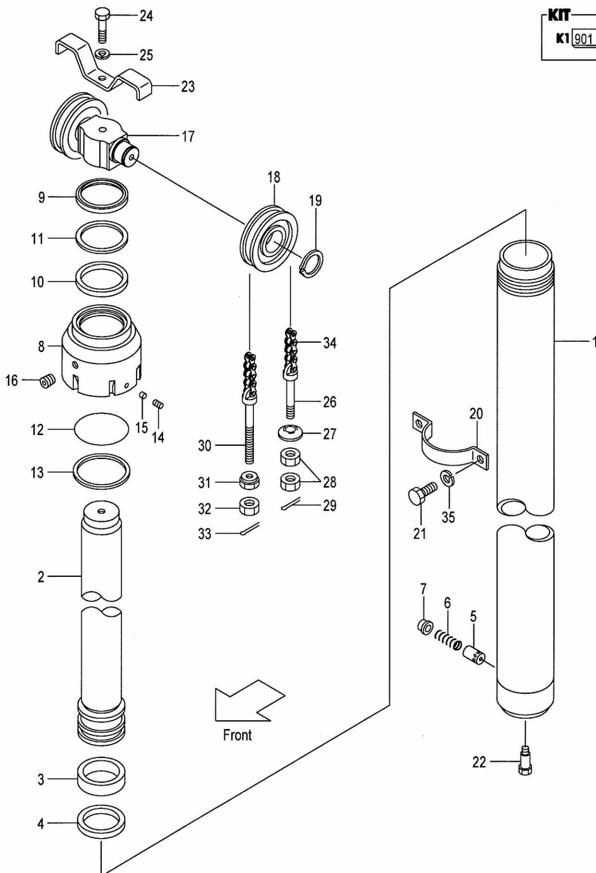
FIG.190 LIFT CYLINDER(FRONT) [VFM2Y5] (M7030510) リフトシリンダ(フロント)
