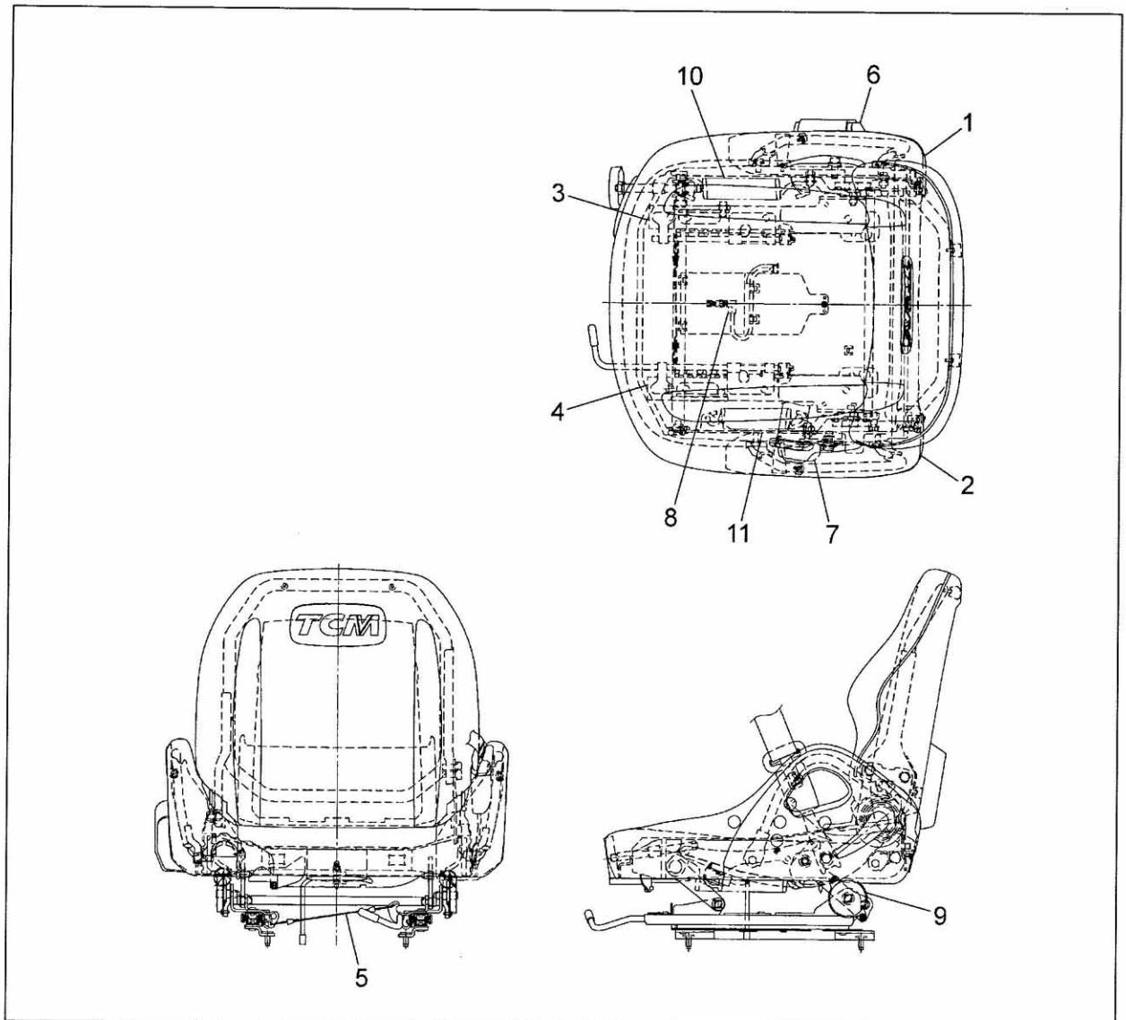
FIG.129A SEAT (F7C36811) シート
