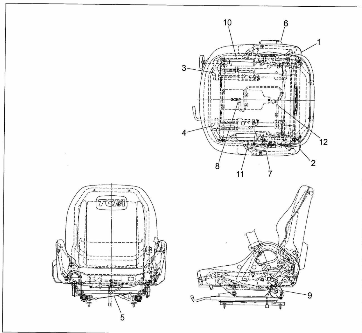
FIG.132 SEAT [OKM] (F7C36840) シート
