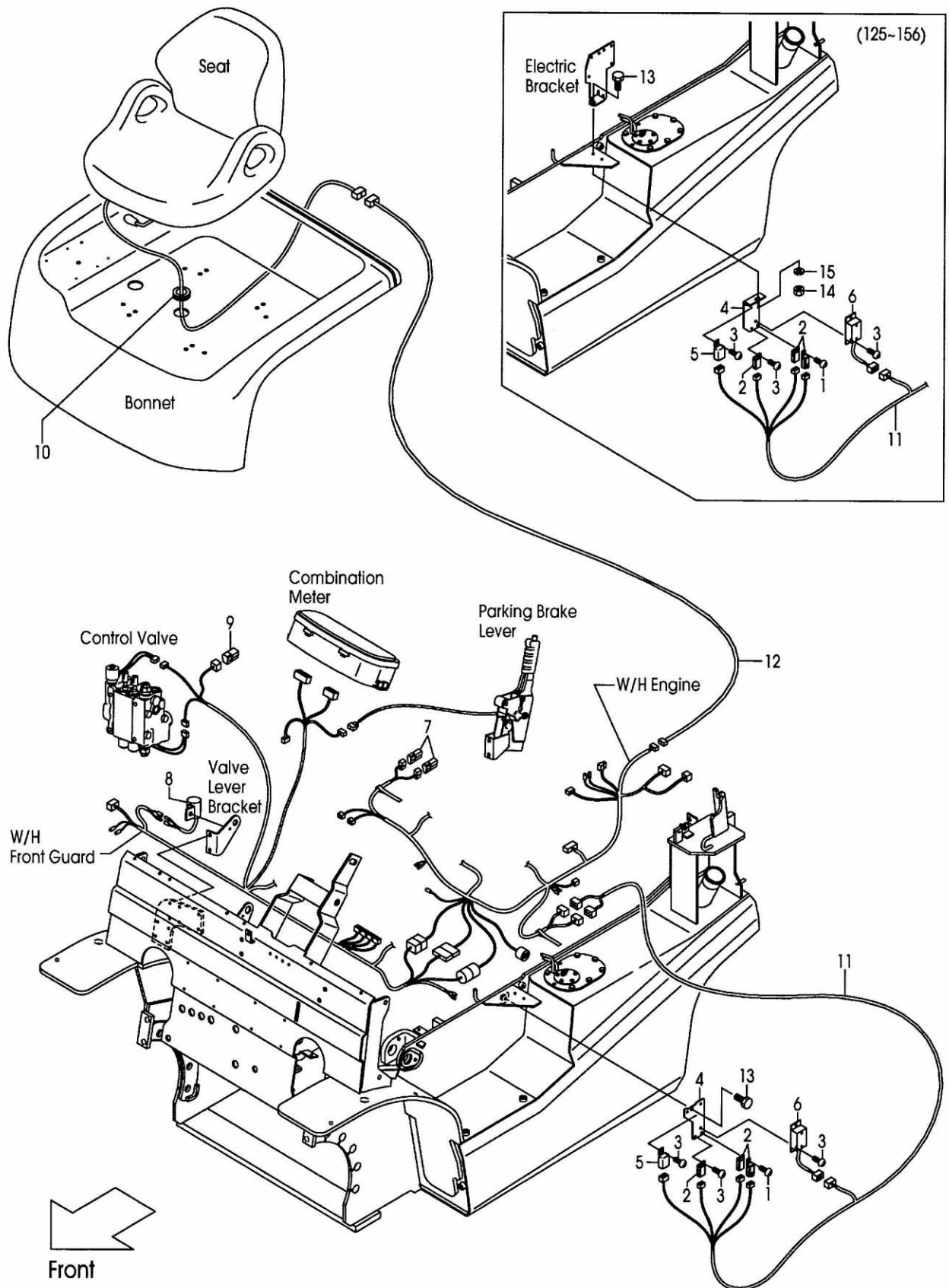
FIG.43A INTERLOCK (F7C32651) インターロック
