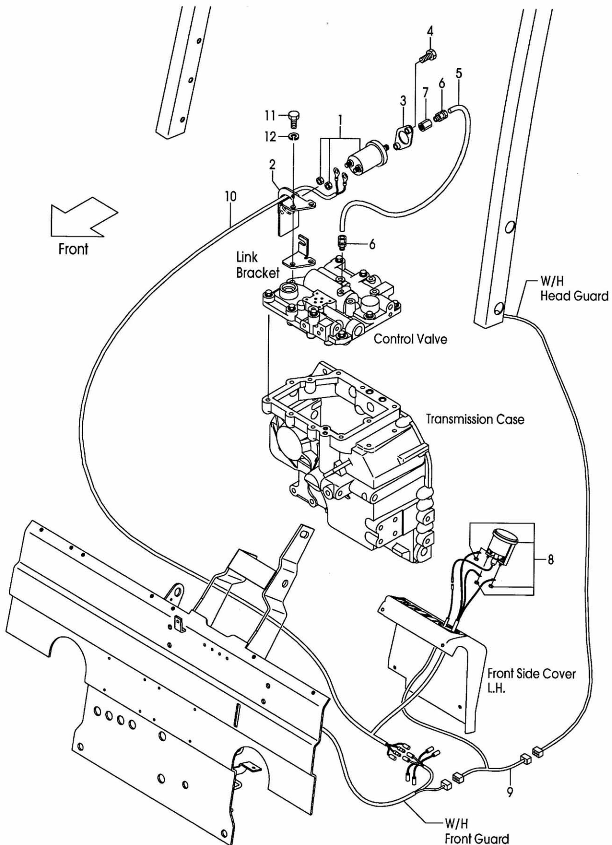
FIG.48 TORQUE CONVERTER PRESSURE METER [TPM] (F7C326D0) トルクコンバータプレッシャメータ
