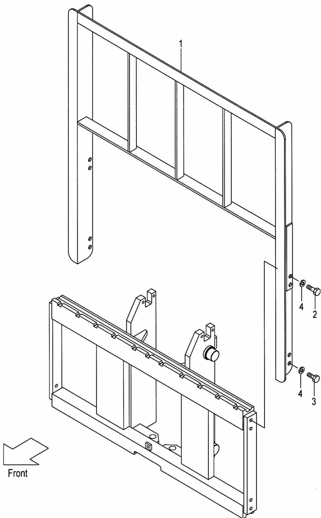
FIG.195 BACKREST [VFHM2Y5] (M7038240) バックレスト
